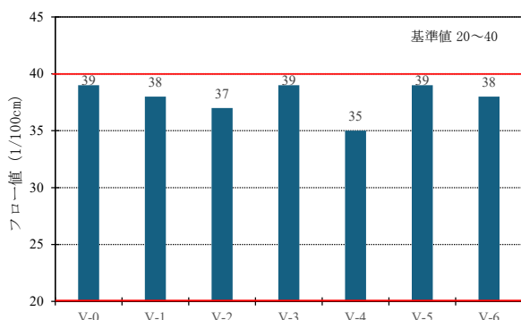
図-3 標準マーシャル安定度試験（フロー値）
