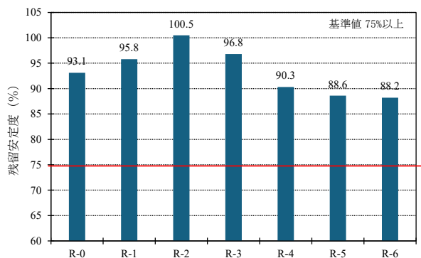
図-12 水浸マーシャル安定度試験（残留安定度）
