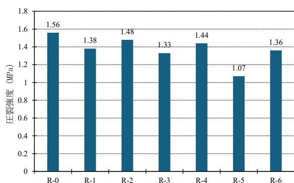
図-17 圧裂試験(圧裂強度)
