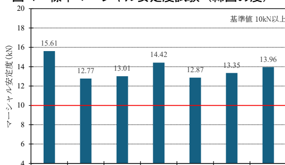
図-2 標準マーシャル安定度試験（安定度）
