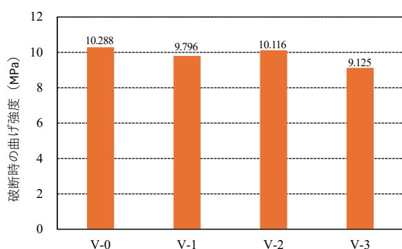
図-44 曲げ試験（強度）
