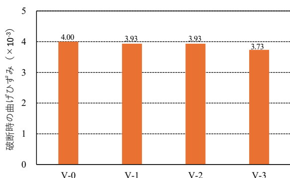
図-45 曲げ試験（破断時のひずみ）
