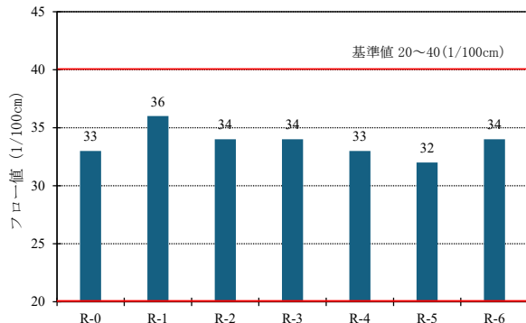
図-11 標準マーシャル安定度試験（フロー値）
