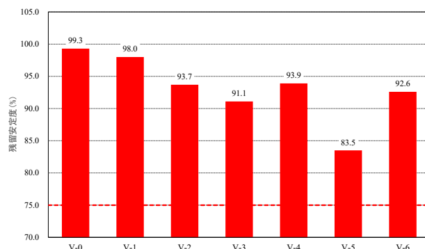
図-23 水浸マーシャル安定度試験（残留安定度）
