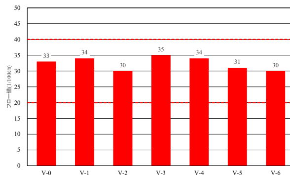
図-22 標準マーシャル安定度試験（フロー値）
