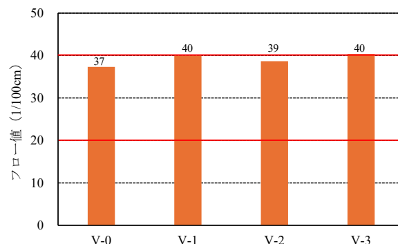
図-41 標準マーシャル安定度試験（フロー値）
