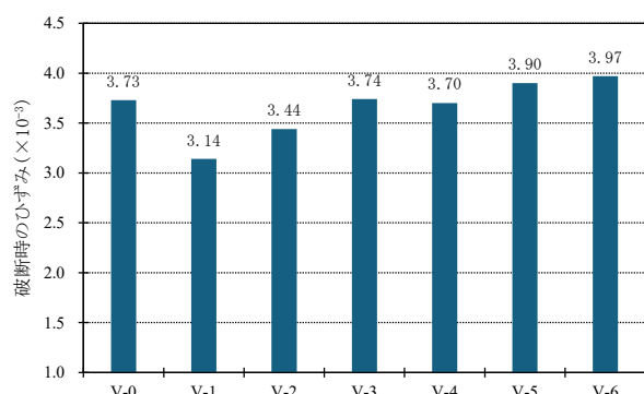
図-7 曲げ試験（破断時のひずみ）
