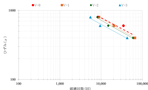
図-46 曲げ疲労試験
