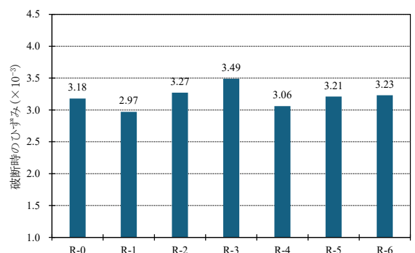
図-15 曲げ試験（破断時のひずみ）
