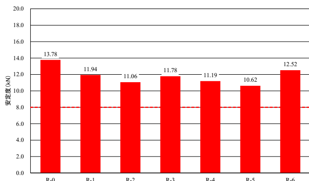
図-29 標準マーシャル安定度試験（安定度）
