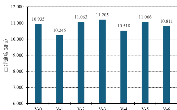
図-6 曲げ試験（強度）
