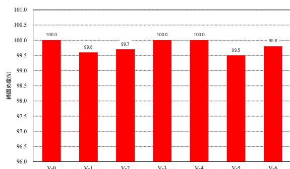
図-20 標準マーシャル安定度試験（締固め度）
