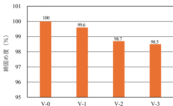
図-39 標準マーシャル安定度試験（締固め度）
