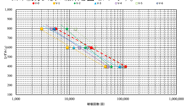
図-27 曲げ疲労試験
