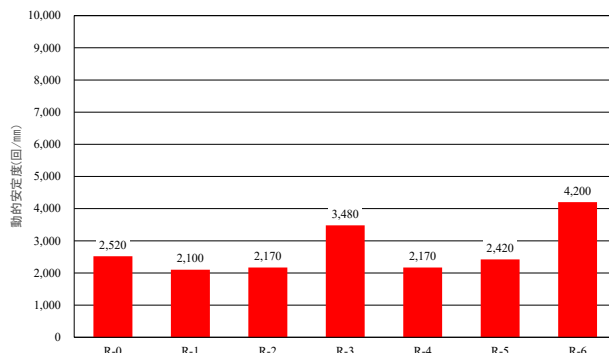
図-32 ホイールトラッキング試験（動的安定度）
