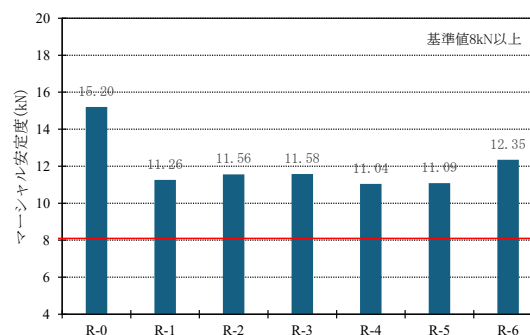
図-10 標準マーシャル安定度試験（安定度）
