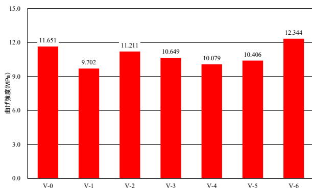
図-25 曲げ試験（強度）
