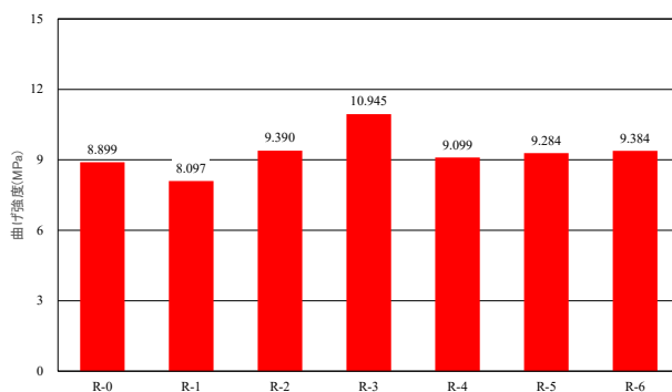
図-33 曲げ試験（強度）
