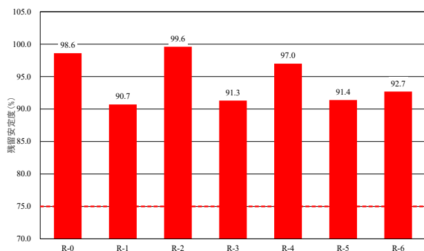
図-31 水浸マーシャル安定度試験（残留安定度）
