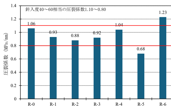
図-19 圧裂試験(圧裂係数)
