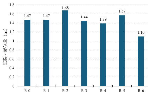
図-18 圧裂試験(変位量)
