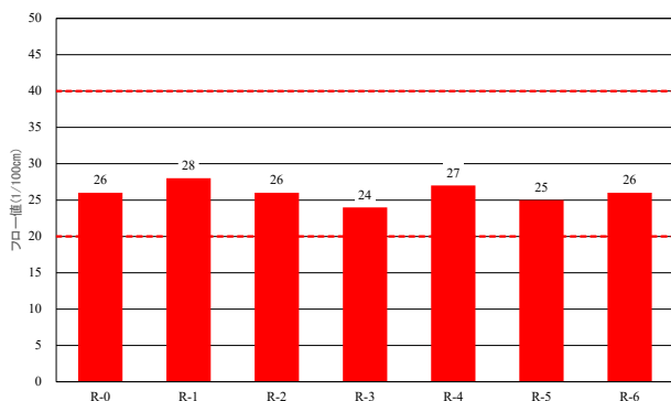
図-30 標準マーシャル安定度試験（フロー値）
