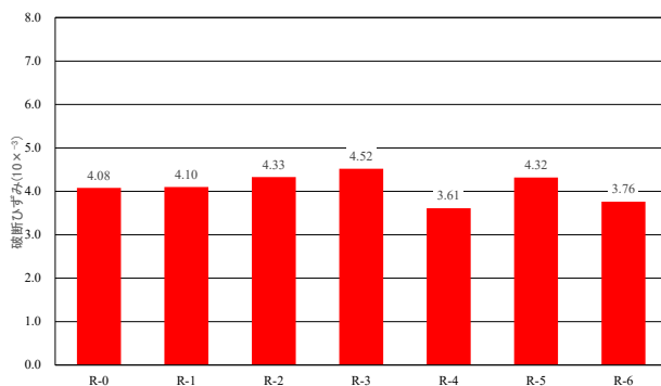
図-34 曲げ試験（破断時のひずみ）
