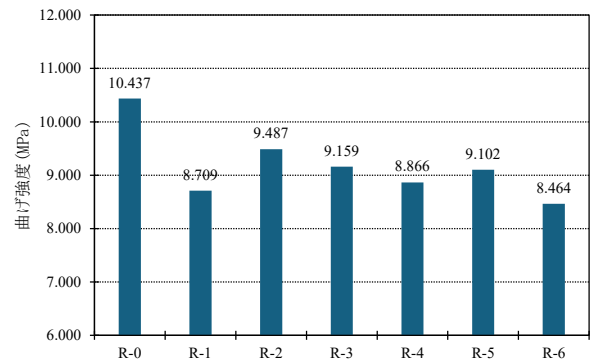
図-14 曲げ試験（強度）
