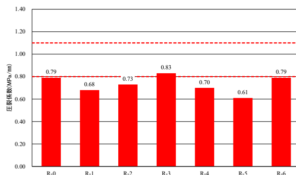
図-38 圧裂試験 (圧裂係数)
