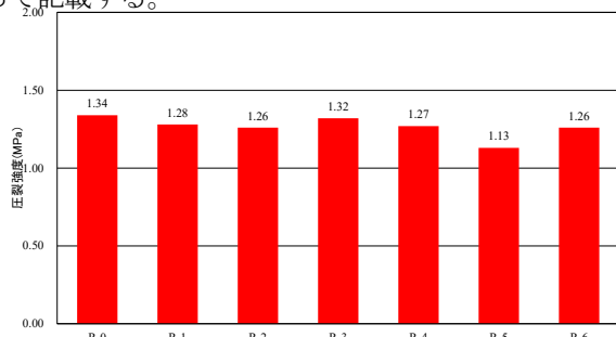
図-36 圧裂試験 (圧裂強度)
