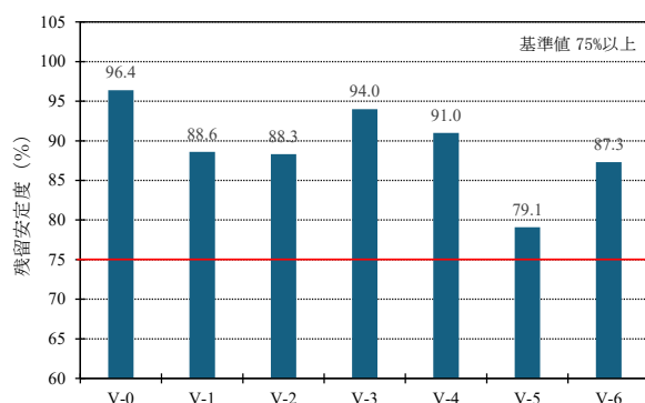
図-4 水浸マーシャル安定度試験（残留安定度）
