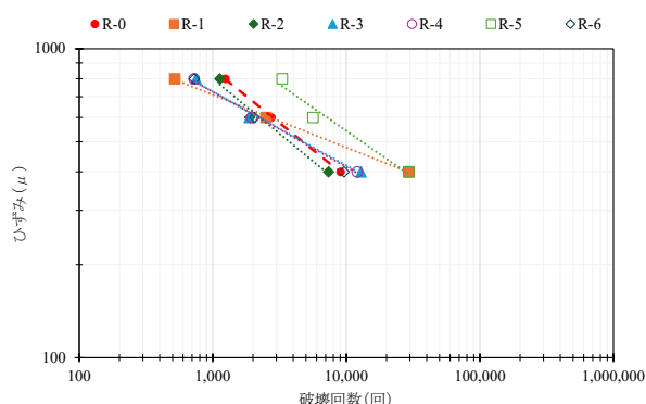
図-16 曲げ疲労試験
