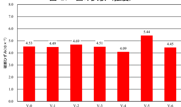
図-26 曲げ試験（破断時のひずみ）
