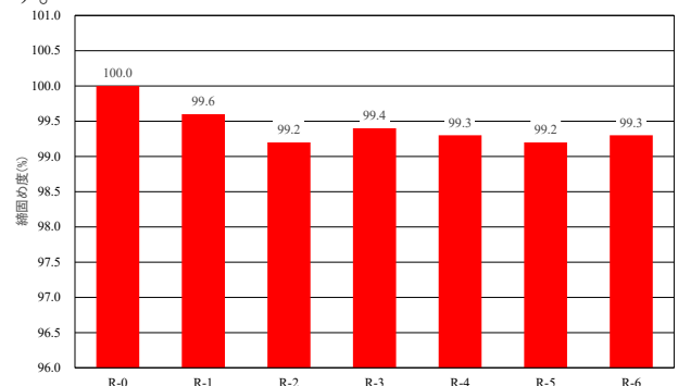
図-28 標準マーシャル安定度試験（締固め度）
