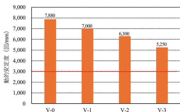
図-43 ホイールトラッキング試験（動的安定度）
