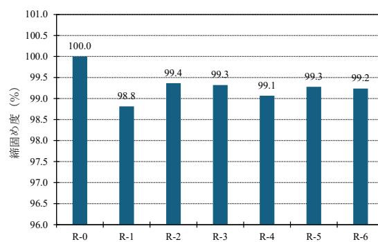
図-9 標準マーシャル安定度試験（締固め度）
