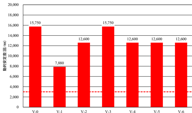
図-24 ホイールトラッキング試験（動的安定度）
