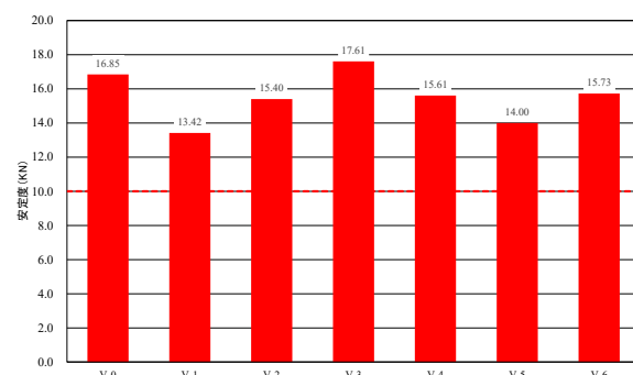
図-21 標準マーシャル安定度試験（安定度）
