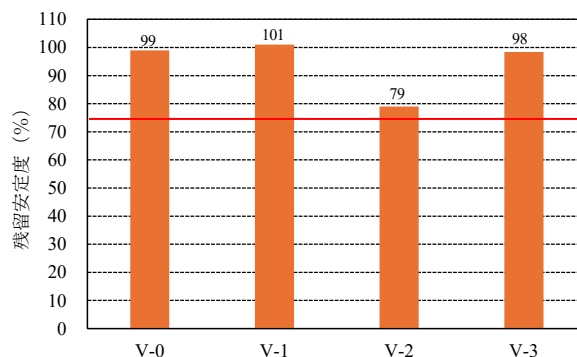
図-42 水浸マーシャル安定度試験（残留安定度）
