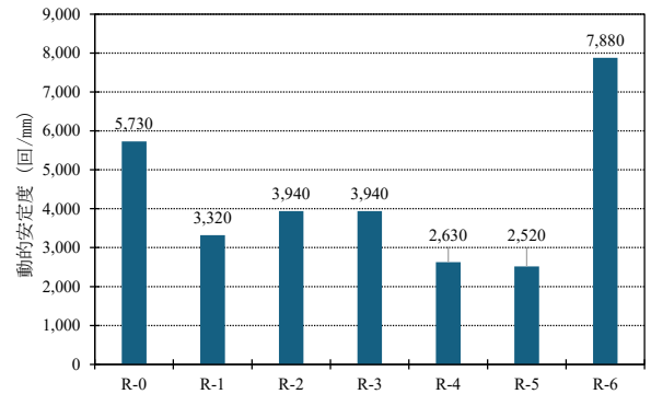
図-13 ホイールトラッキング試験（動的安定度）
