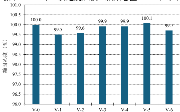
図-1 標準マーシャル安定度試験（縮固め度）
