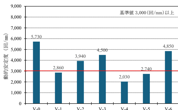
図-5 ホイールトラッキング試験（動的安定度）
