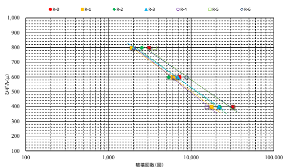
図-35 曲げ疲労試験
