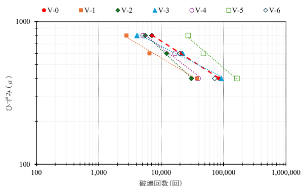
図-8 曲げ疲労試験
