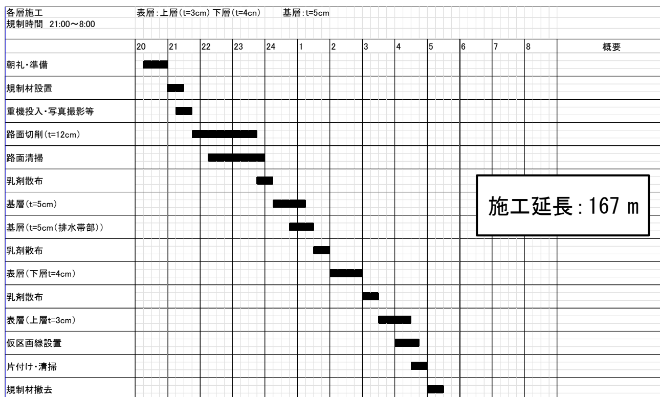
図3 各層施工の施工時間割（案）
