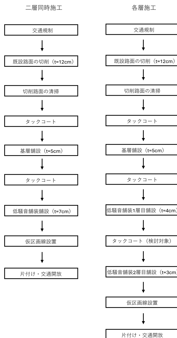
図1 施工フロー
