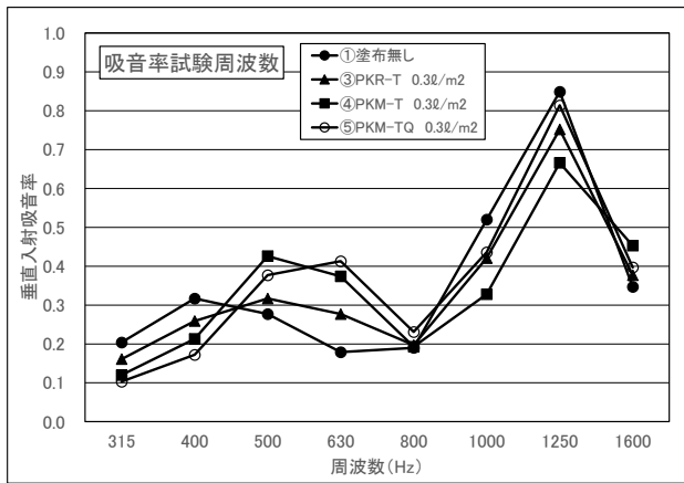
図 11 垂直入射吸音率(乳剤塗布 0.3L/m² との比較)
