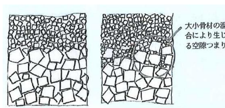
図 9 締固め効果が高くなった場合の断面構造の違い
