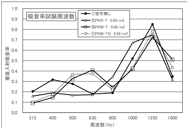
図 12 垂直入射吸音率(乳剤塗布 0.6L/m² との比較)
