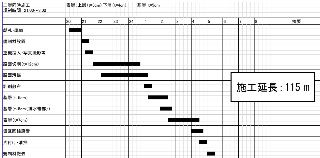
図2 二層同時施工の施工時間割（案）
