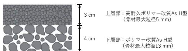
図4 供試体模式図
