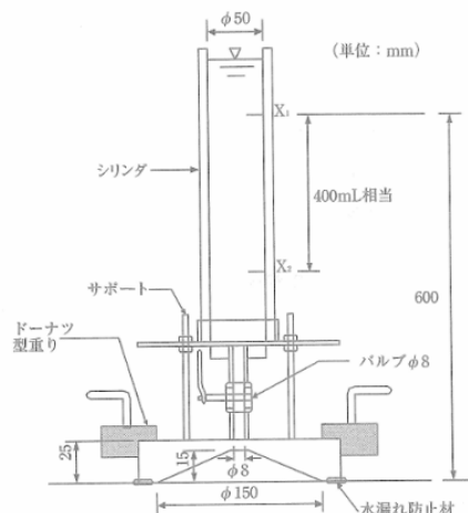
図5 透水試験模式図
