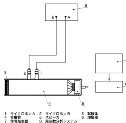
図7 垂直入射吸音率試験模式図
