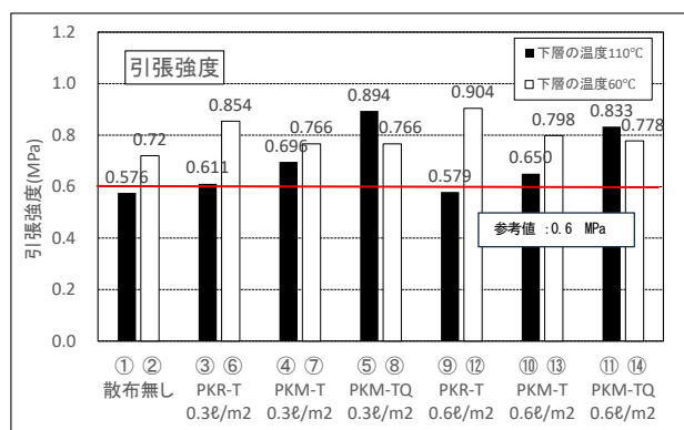
図15 引張強度試験結果
