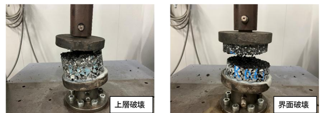
写真 2 PKR-T 0.6L/m²(下層温度条件: 左 110℃・右 60℃)
