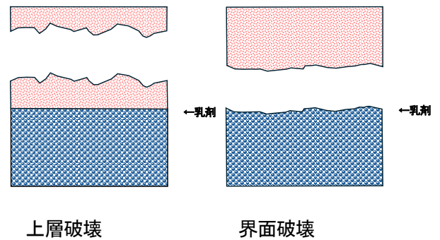
図 14 上層破壊及び界面破壊の模式図
