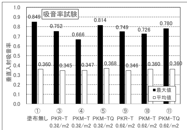
図 13 垂直入射吸音率(最大値と平均値)
