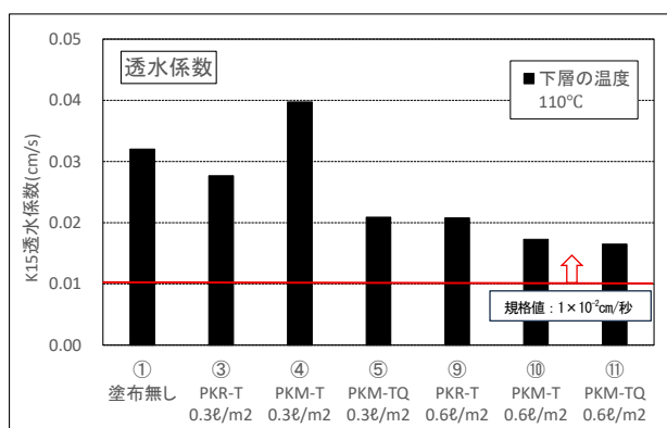
図 10 透水試験結果
