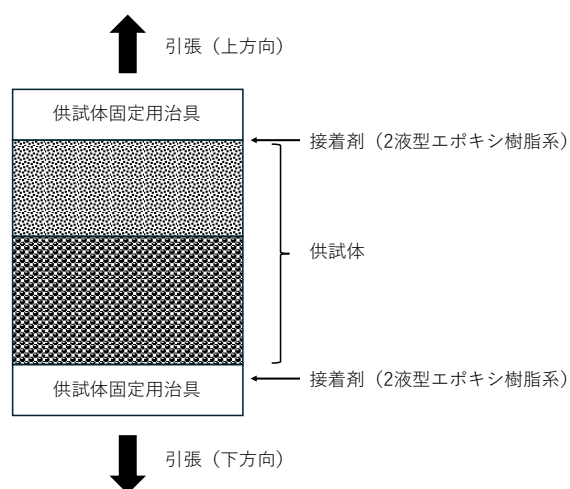
図6 引張試験模式図
