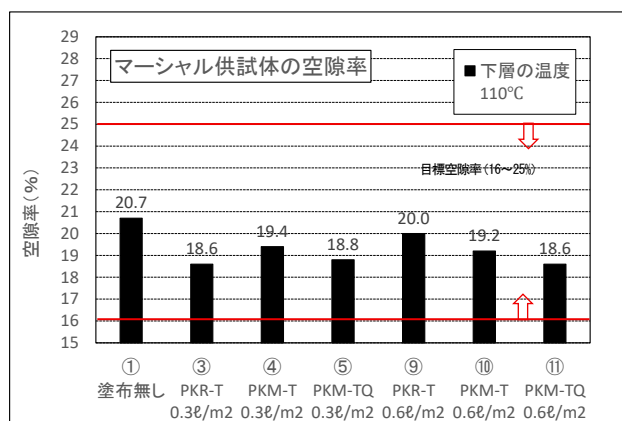
図 8 空隙率測定結果
