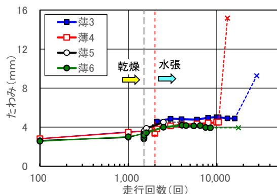
図-12 たわみの推移
