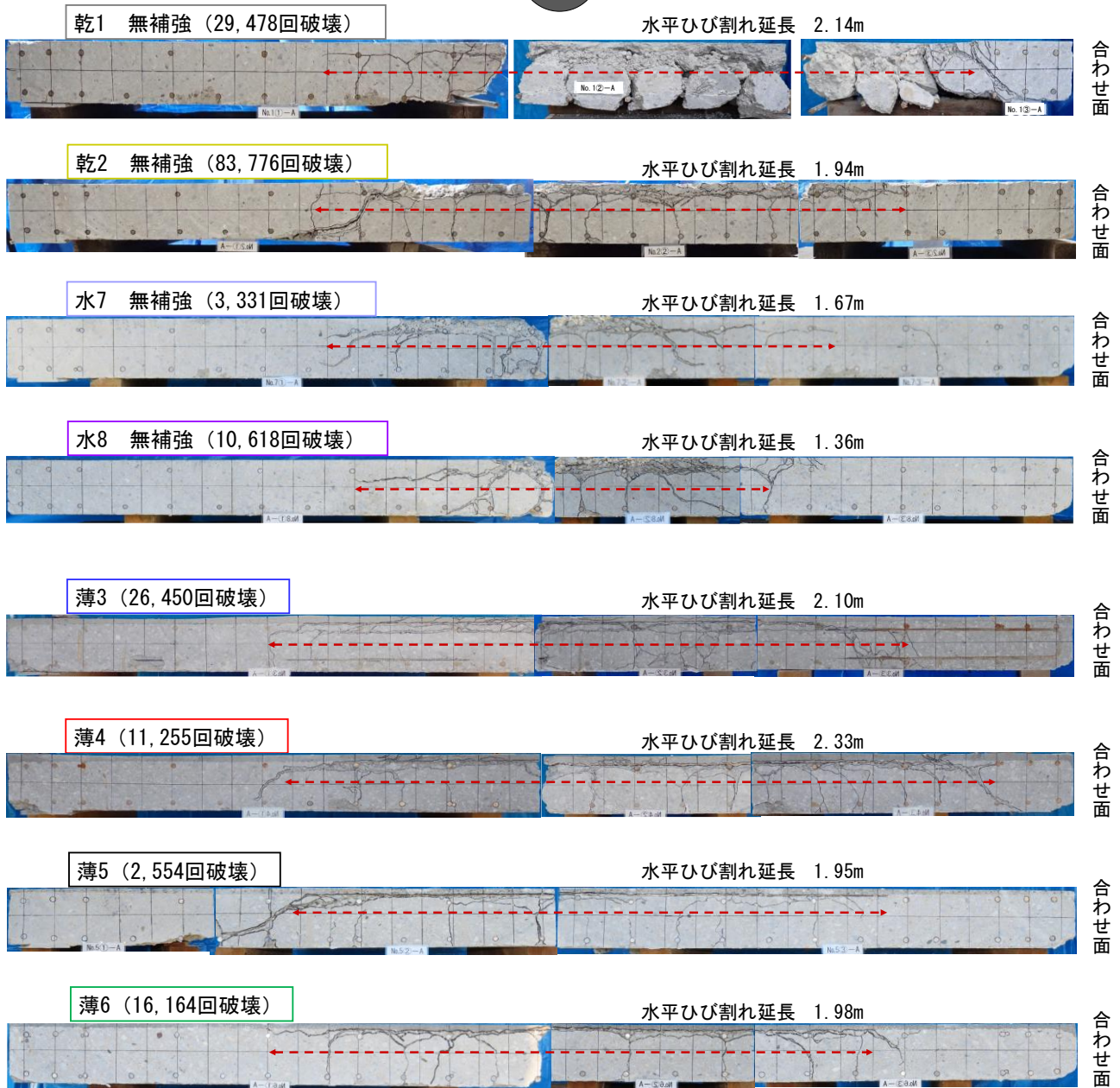
写真-12 橋軸方向の切断面
