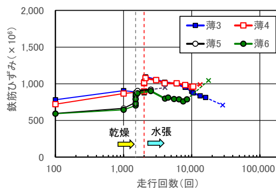
図-14 下側配力鉄筋ひずみの推移
