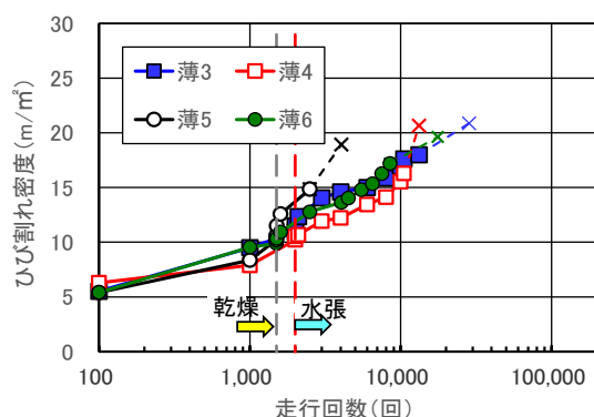
図-17 下面ひび割れ密度の推移
