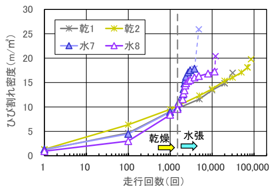
図-11 下面ひび割れ密度の推移
