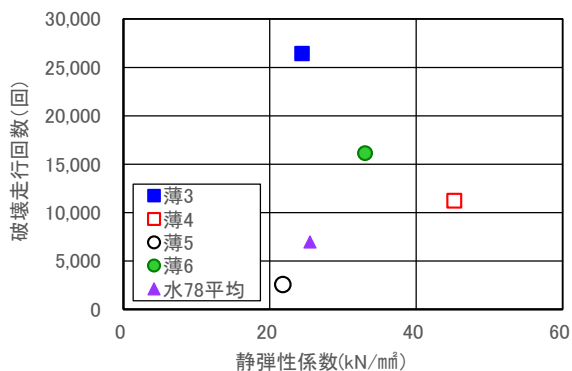
図-19 静弾性係数と破壊走行回数
