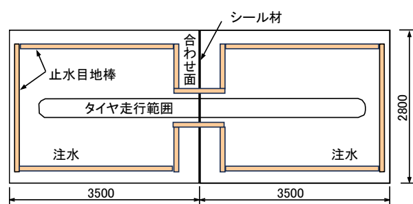
図-3 水張条件の水張の方法
