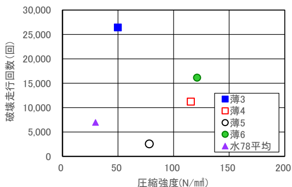
図-18 圧縮強度と破壊走行回数
