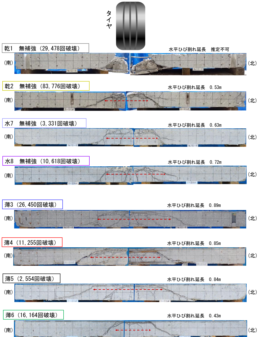
写真－11 橋軸直角方向の切断面
