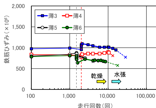
図-13 下側主鉄筋ひずみの推移
