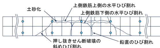
図-27 ひび割れの模式図(橋軸直角方向)
