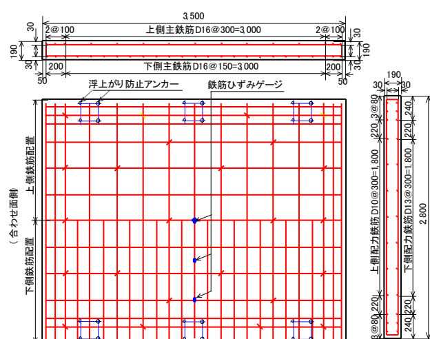
図-4 床版試験体の形状寸法（母材）
