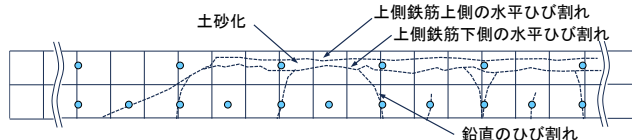
図-28 ひび割れの模式図(橋軸方向)
