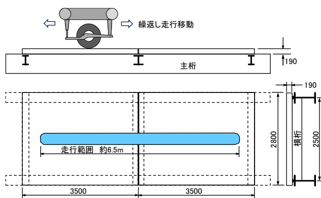
図-2 床版試験体設置図
