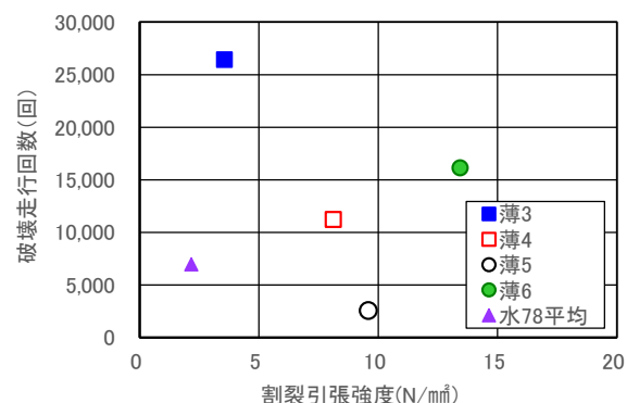
図-21 割裂引張強度と破壊走行回数
