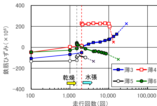
図-15 上側主鉄筋ひずみの推移
