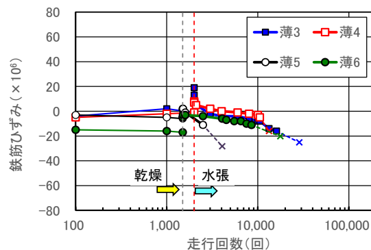
図-16 上側配力鉄筋ひずみの推移
