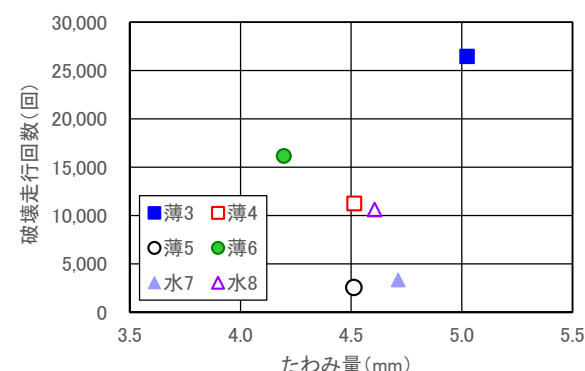
図-23 たわみ量と破壊走行回数
