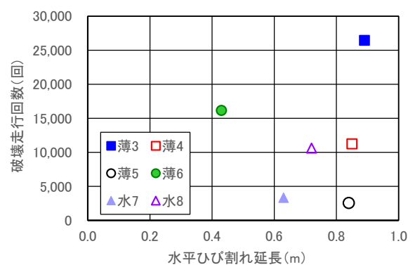
図-26 水平ひび割れの延長と破壊走行回数 (橋軸直角方向)
