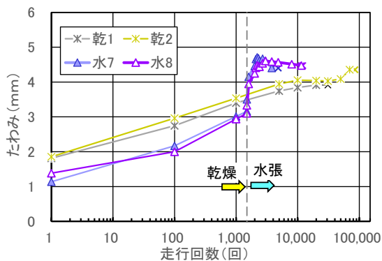
図-5 たわみの推移
