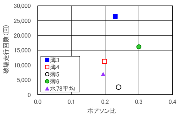
図-20 ポアソン比と破壊走行回数
