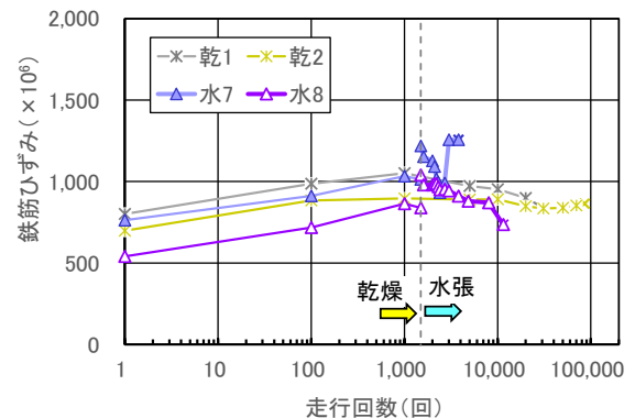
図-7 下側主鉄筋ひずみの推移
