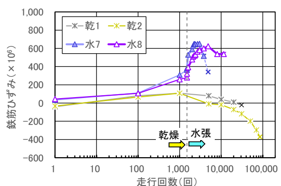
図-10 上側配力鉄筋ひずみの推移
