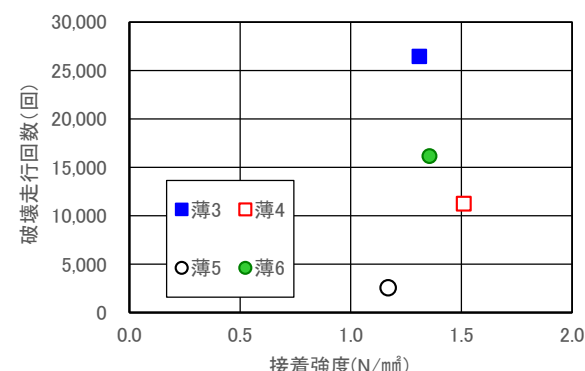
図-22 接着強度と破壊走行回数
