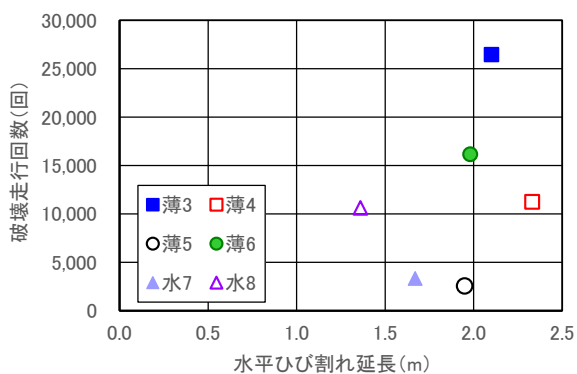
図-25 水平ひび割れの延長と破壊走行回数 (橋軸方向)
