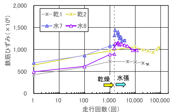
図-8 下側配力鉄筋ひずみの推移
