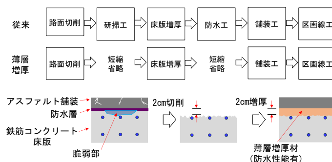
図一 1 薄層増厚工法の概要
