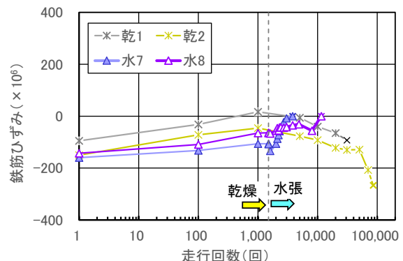
図-9 上側主鉄筋ひずみの推移
