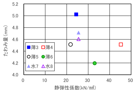
図-24 たわみ量と静弾性係数
