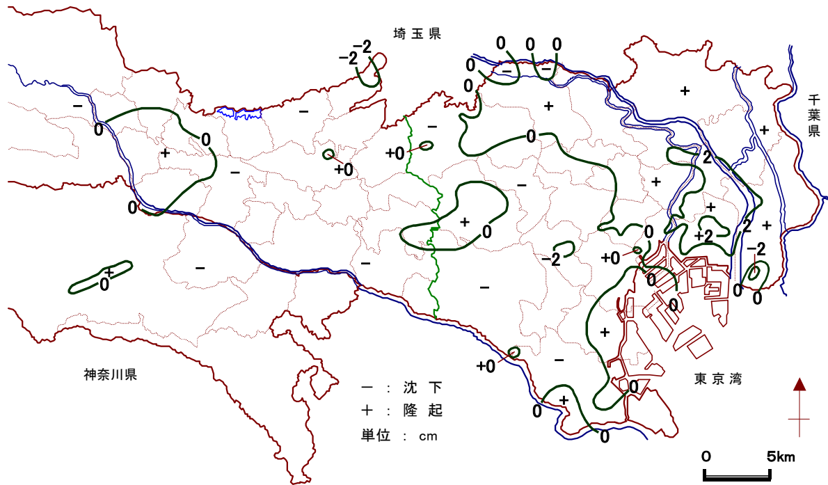
図-3 最近5年間の地盤変動量図（平成14年～平成18年）
