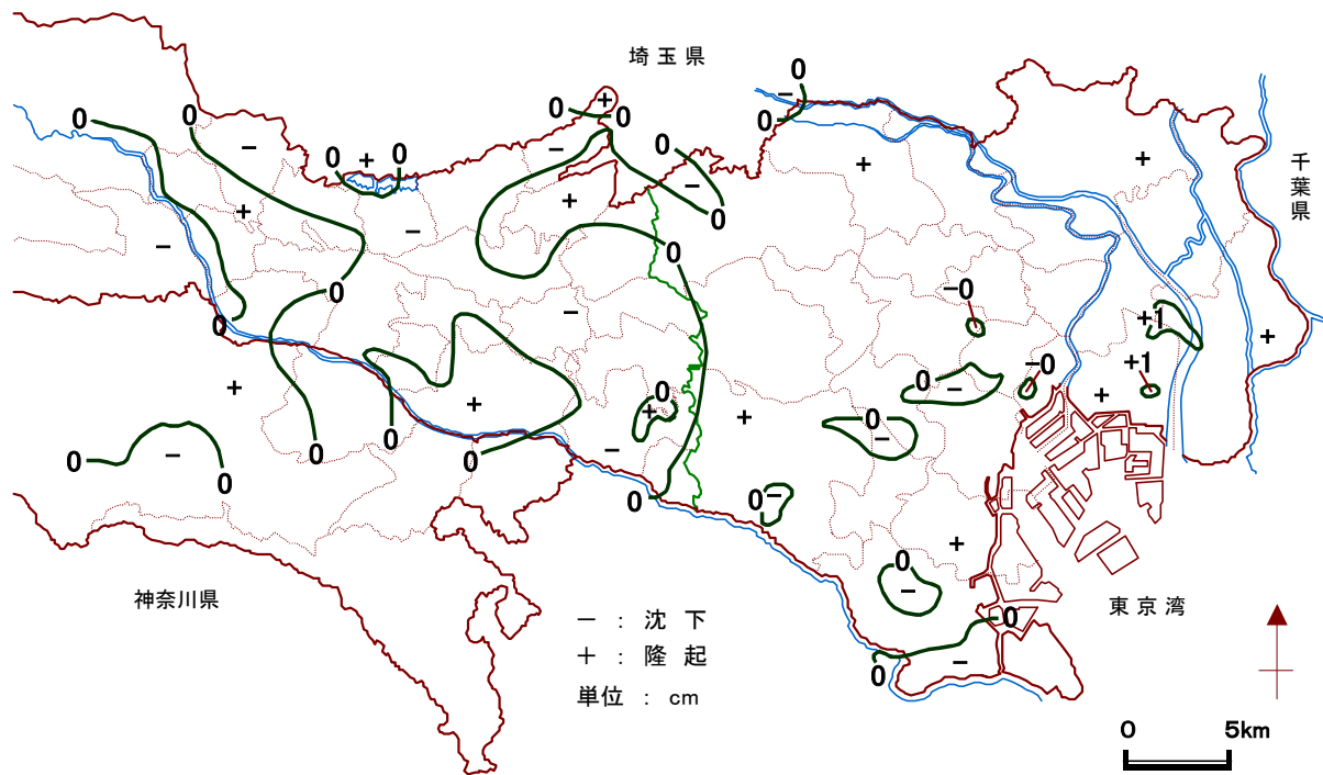
図-2 平成18年の地盤変動量図
