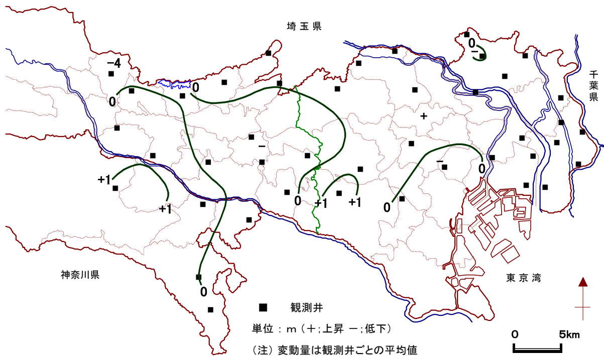
図-6 平成18年の地下水位変動量図
