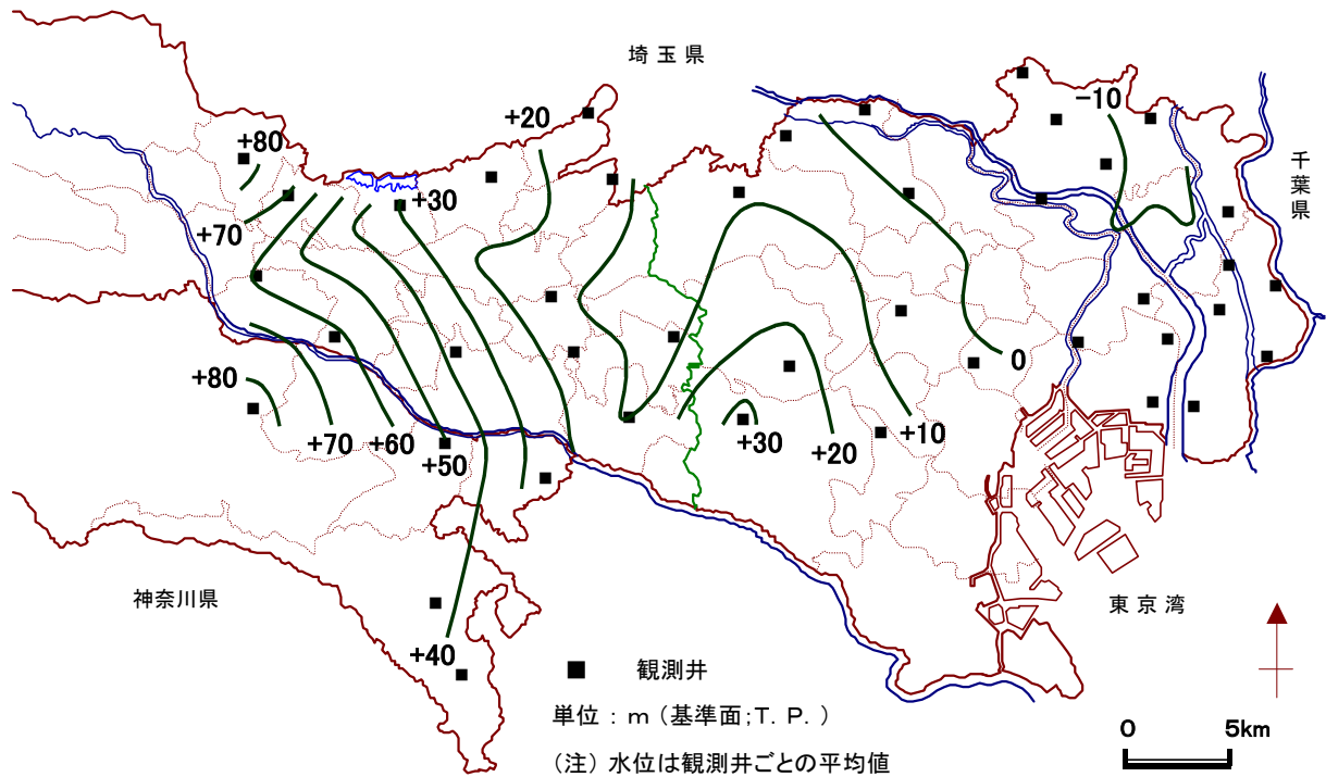
図-5 平成18年末の地下水位等高線図
