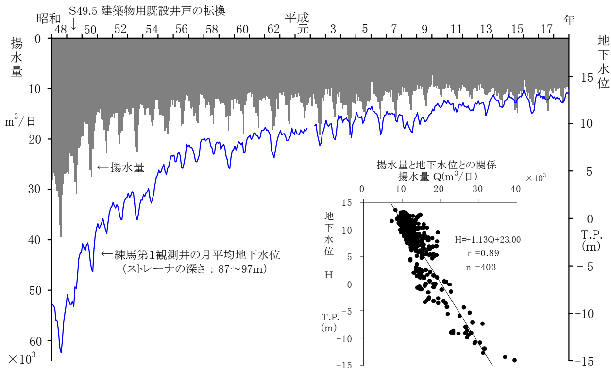
図-14 練馬区内の揚水量と地下水位との関係
