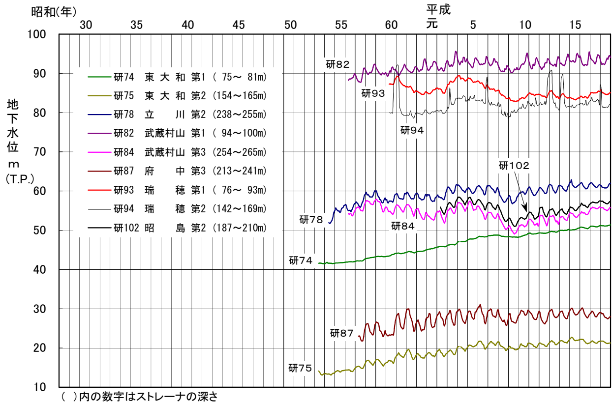
図-12 主な観測井の地下水位変動図（東大和市、武蔵村山市、瑞穂町、昭島市、立川市、府中市）
