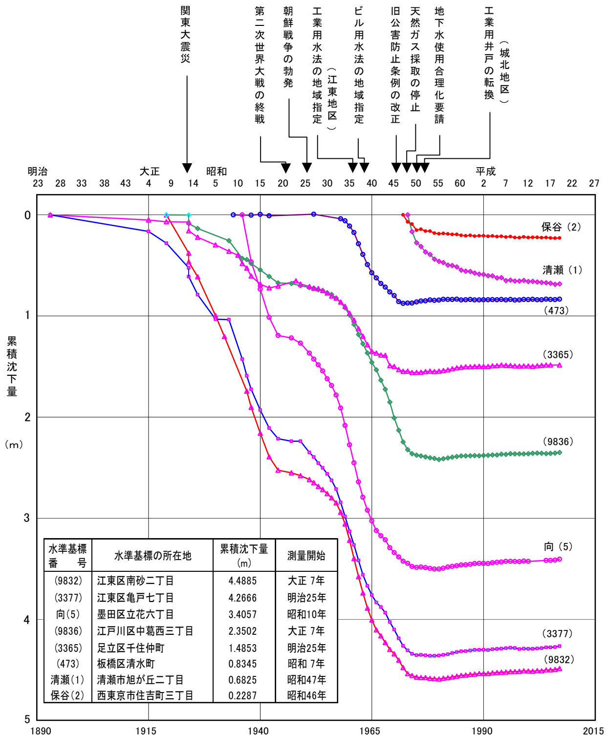
図-15 主要水準基標の累積沈下量図
