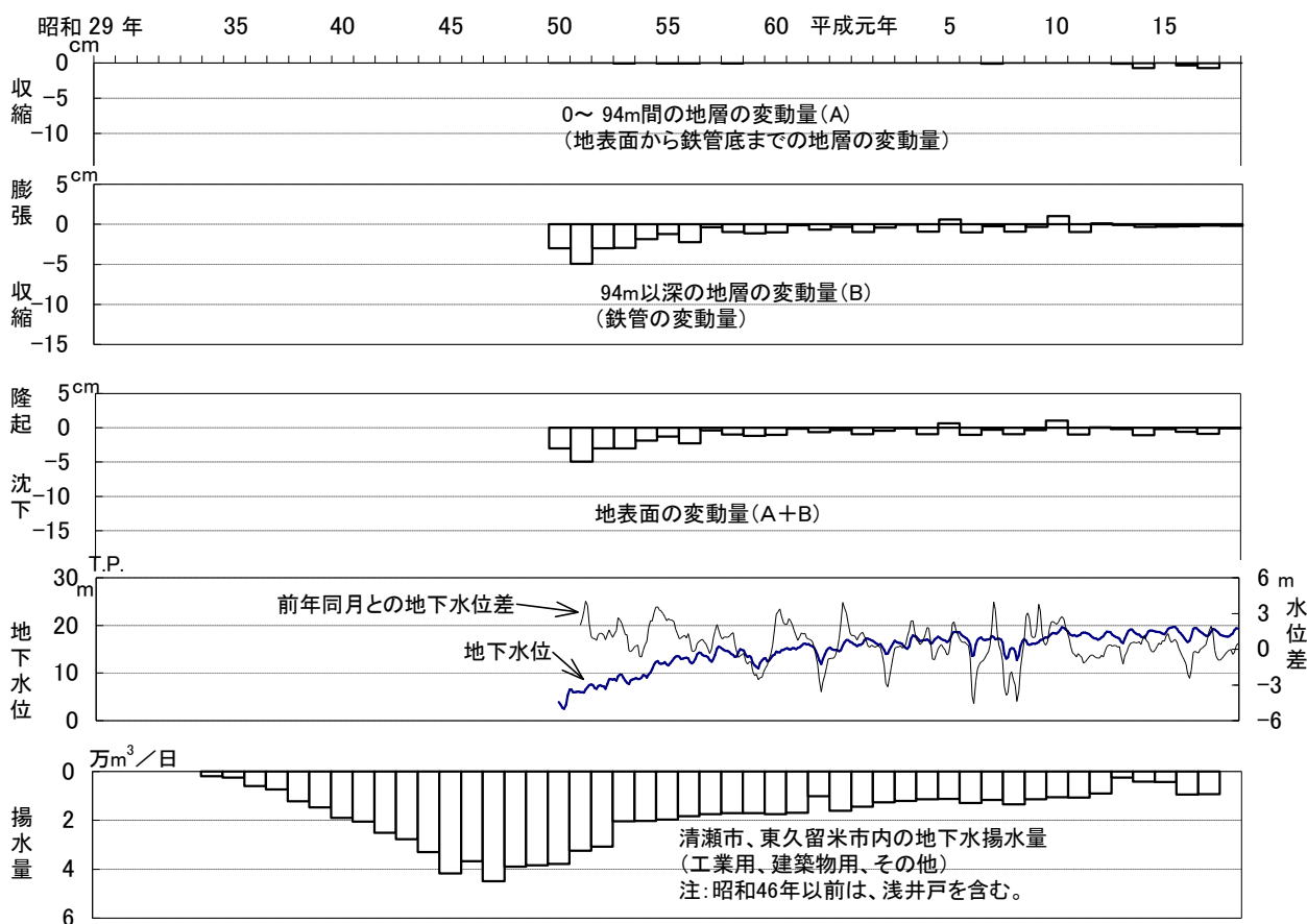
図-20 清瀬第1観測井(94m井)における地盤変動量と地下水位との関係
