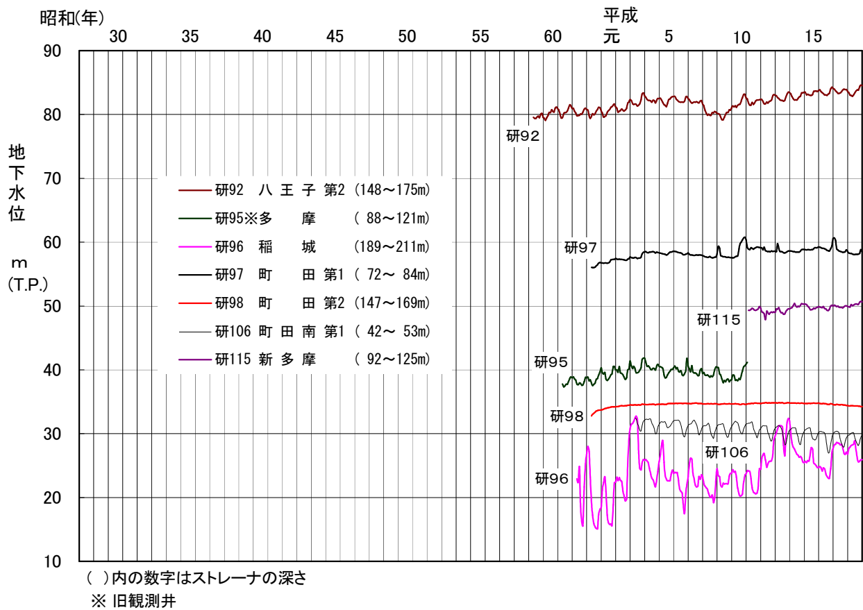
図一13 主な観測井の地下水位変動図（八王子市、多摩市、稲城市、町田市）
