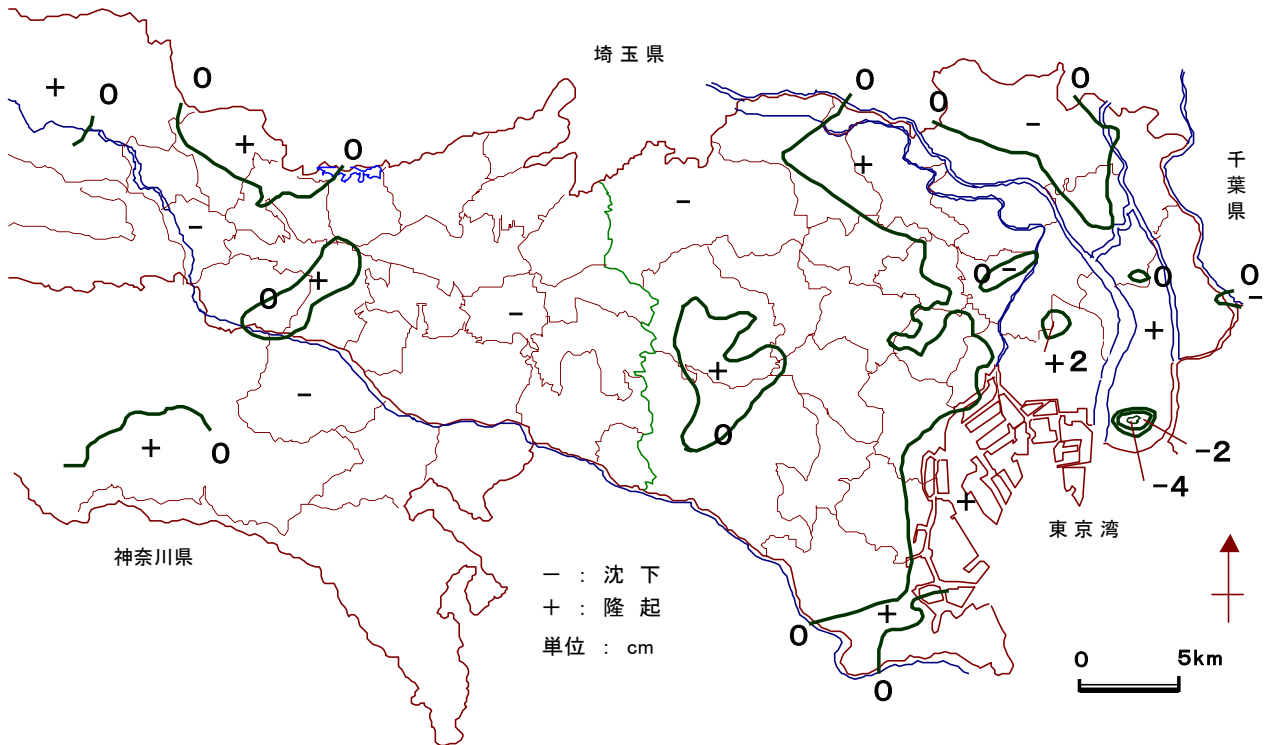
図-3 最近5年間の地盤変動量図（平成12年～平成16年）
