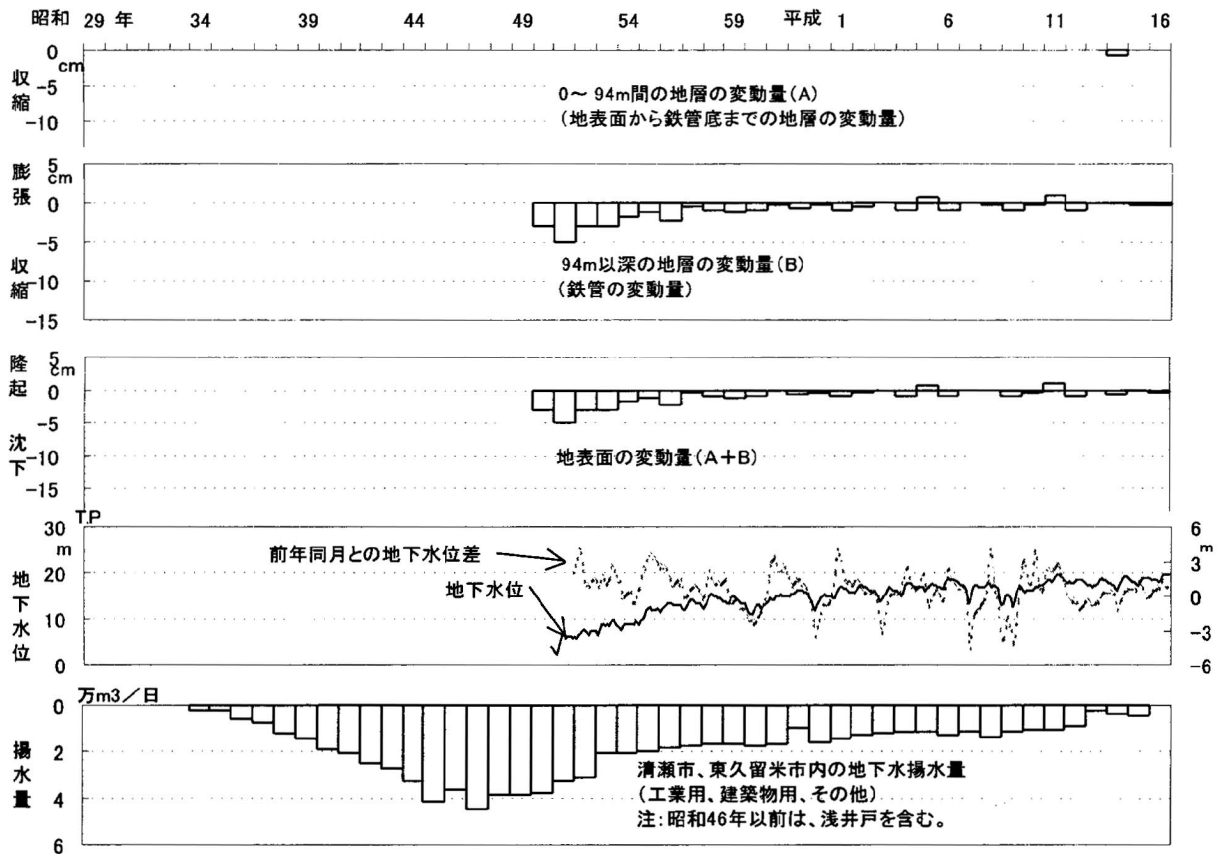
図-27 清瀬第1観測井(94m井)における地盤変動量と地下水位の関係
