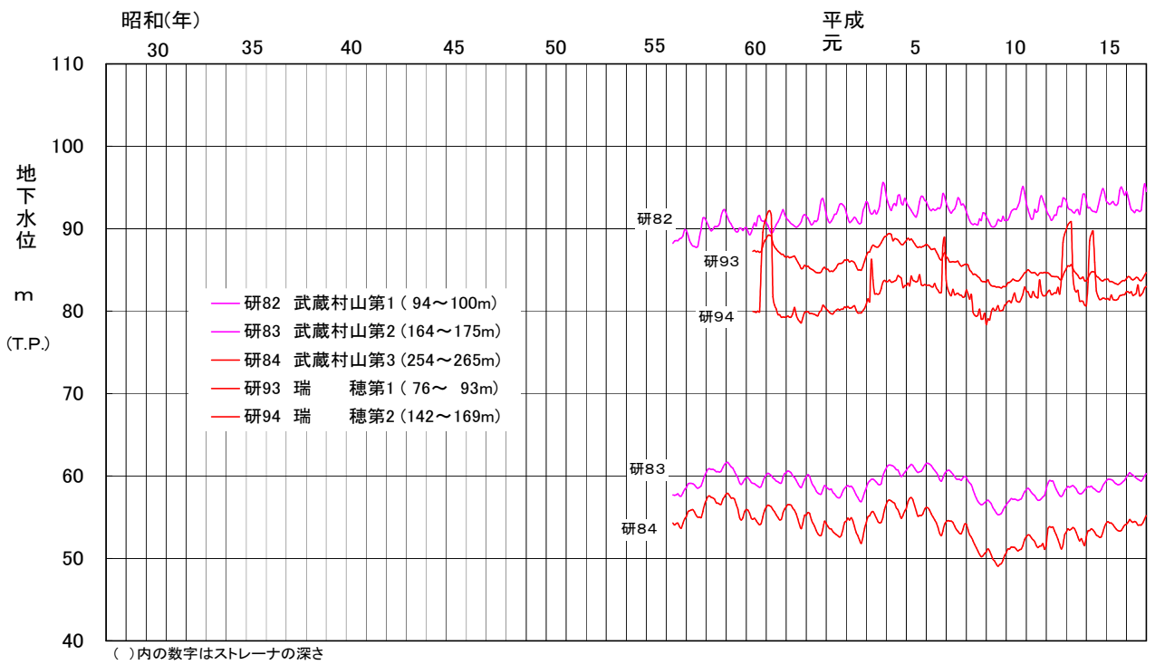
図-16 観測井の地下水位変動図（武蔵村山市、瑞穂町）
