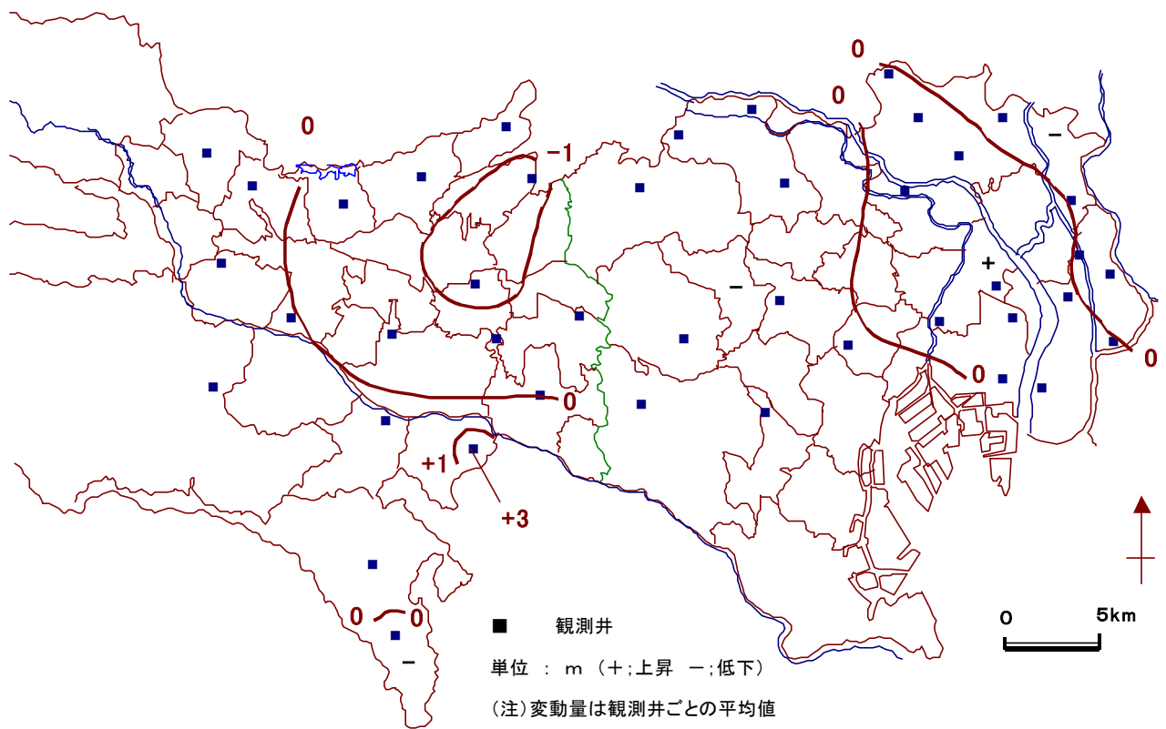
図-6 平成16年の地下水位変動量図
