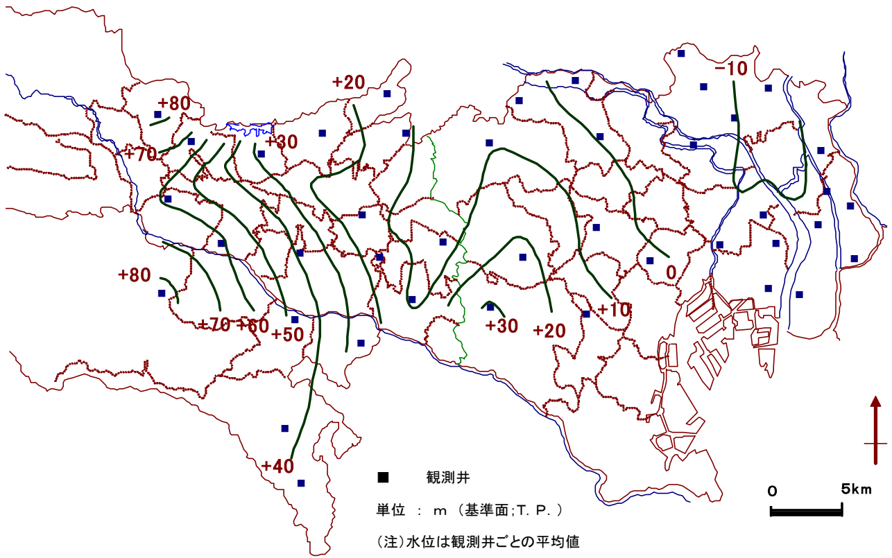
図-5 平成16年末の地下水位等高線図
