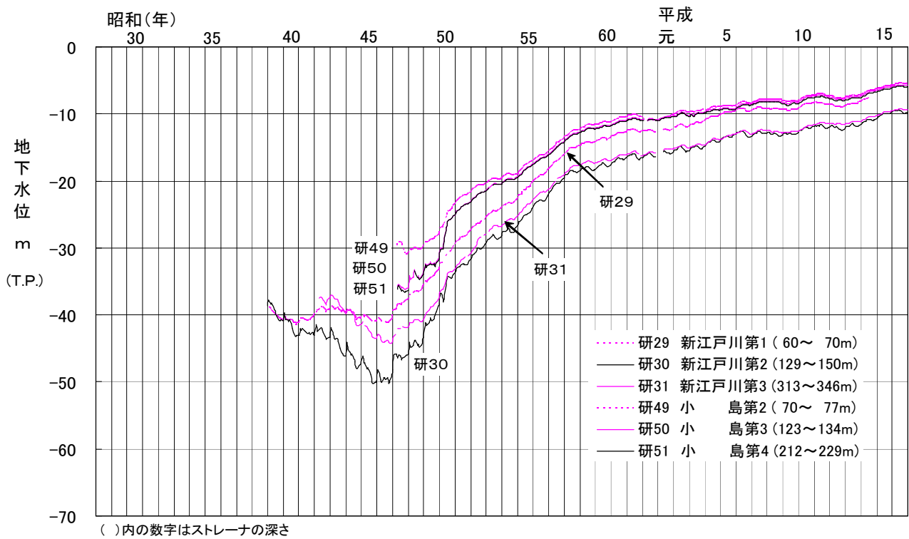
図-8 観測井の地下水水位変動図 (江戸川区その1)
