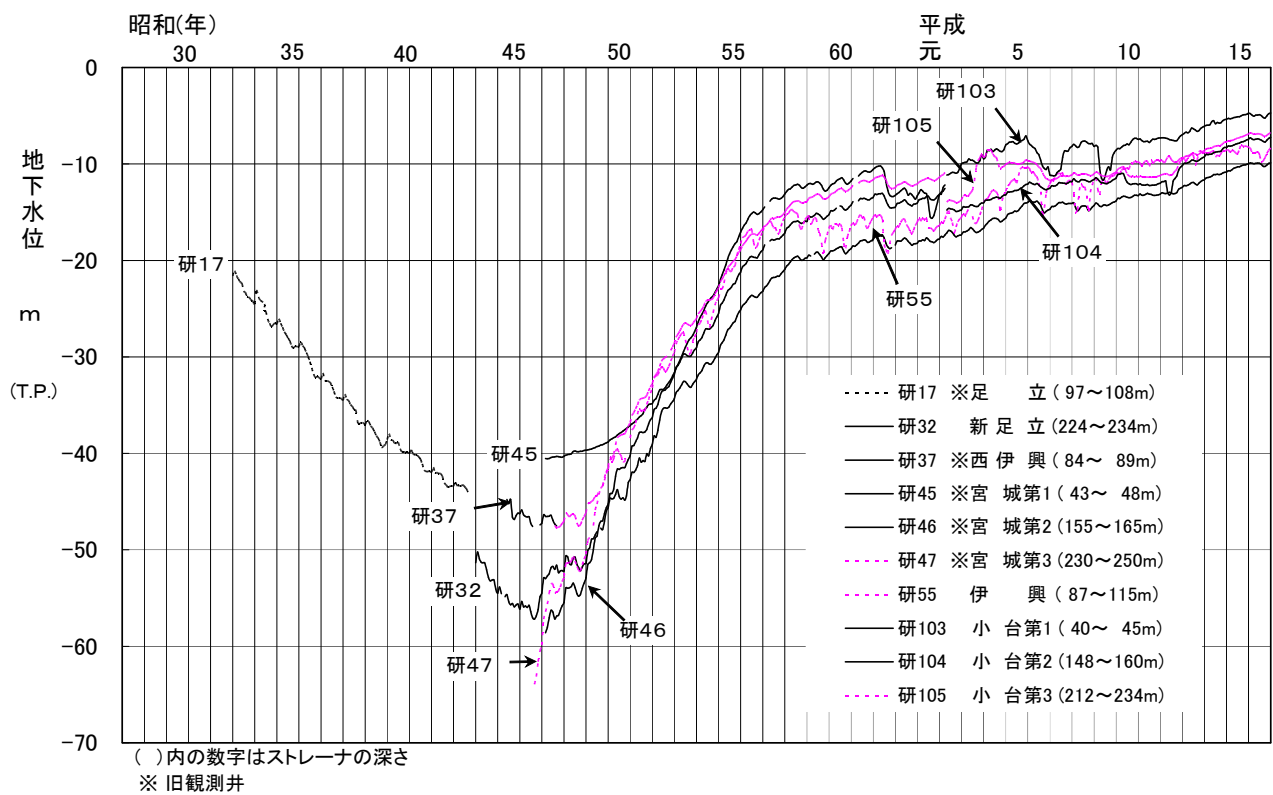
図-10 観測井の地下水位変動図 (足立区その1)
