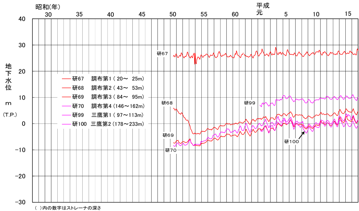
図-17 観測井の地下水水位変動図（調布市、三鷹市）
