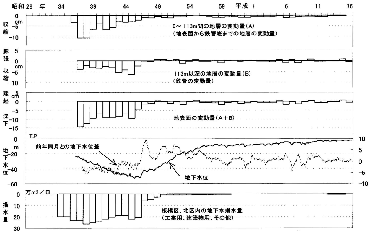
図-25 戸田橋第2観測井(113m井)における地盤変動量と地下水位の関係
