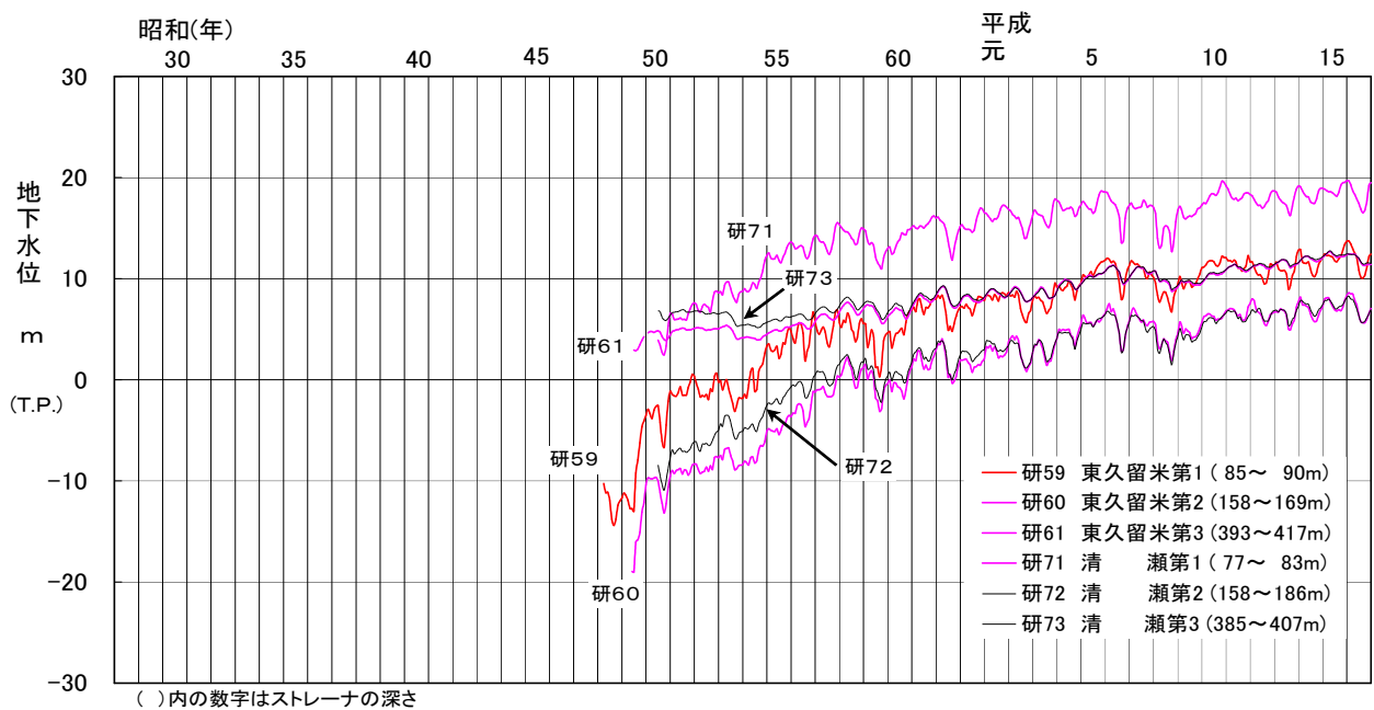
図-14 観測井の地下水位変動図（東久留米市、清瀬市）
