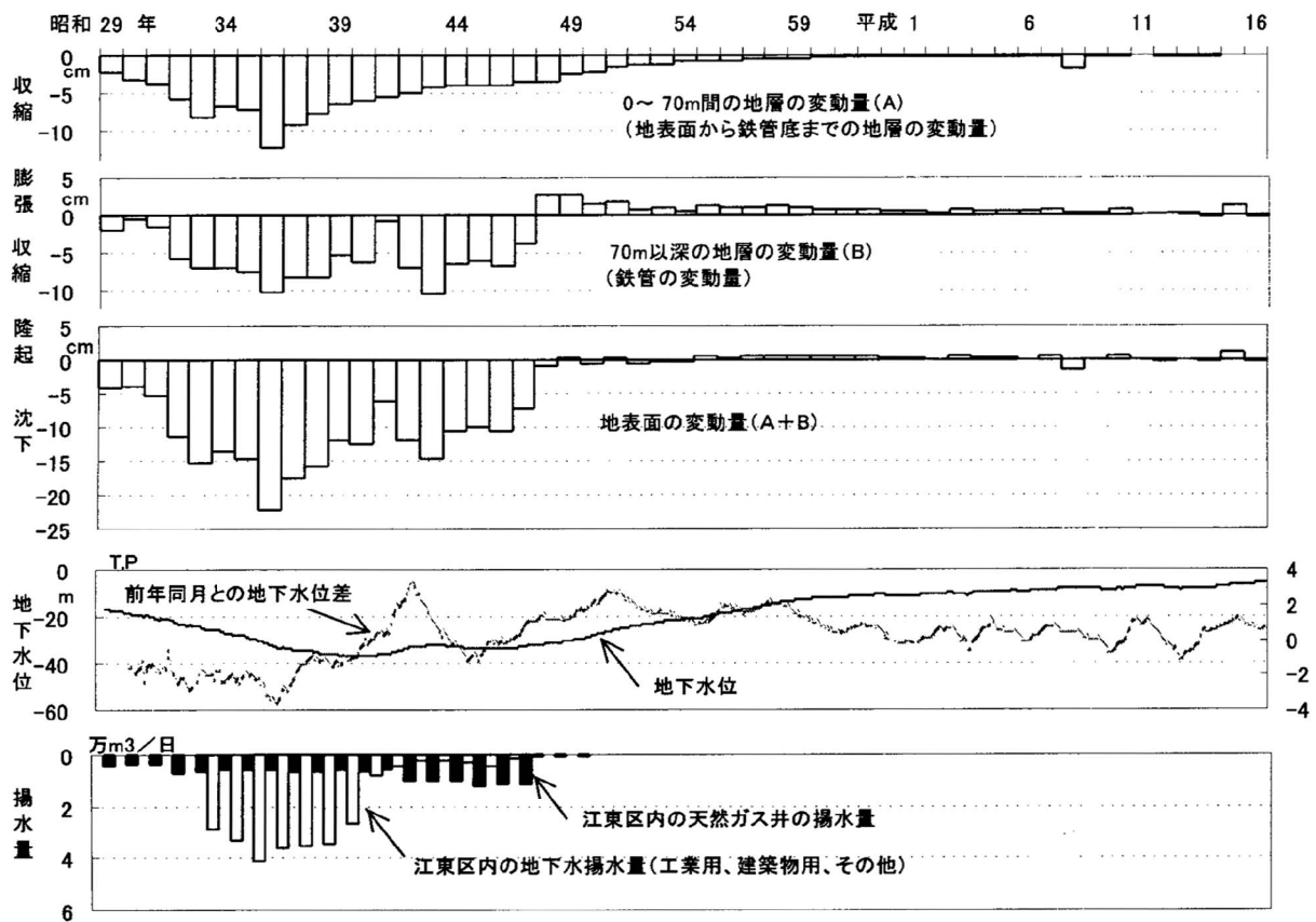
図-24 南砂町第1観測井(70m井)における地盤変動量と地下水位の関係
