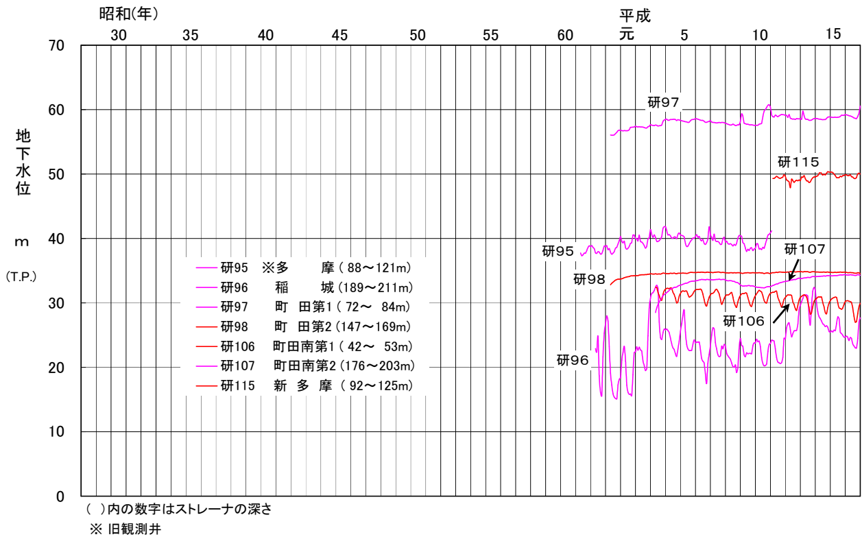
図-20 観測井の地下水水位変動図 (多摩市、稲城市、町田市)
