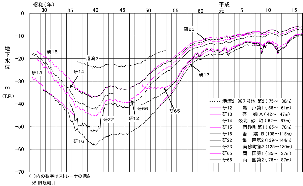
図-7 観測井の地下水水位変動図 (江東区、墨田区)
