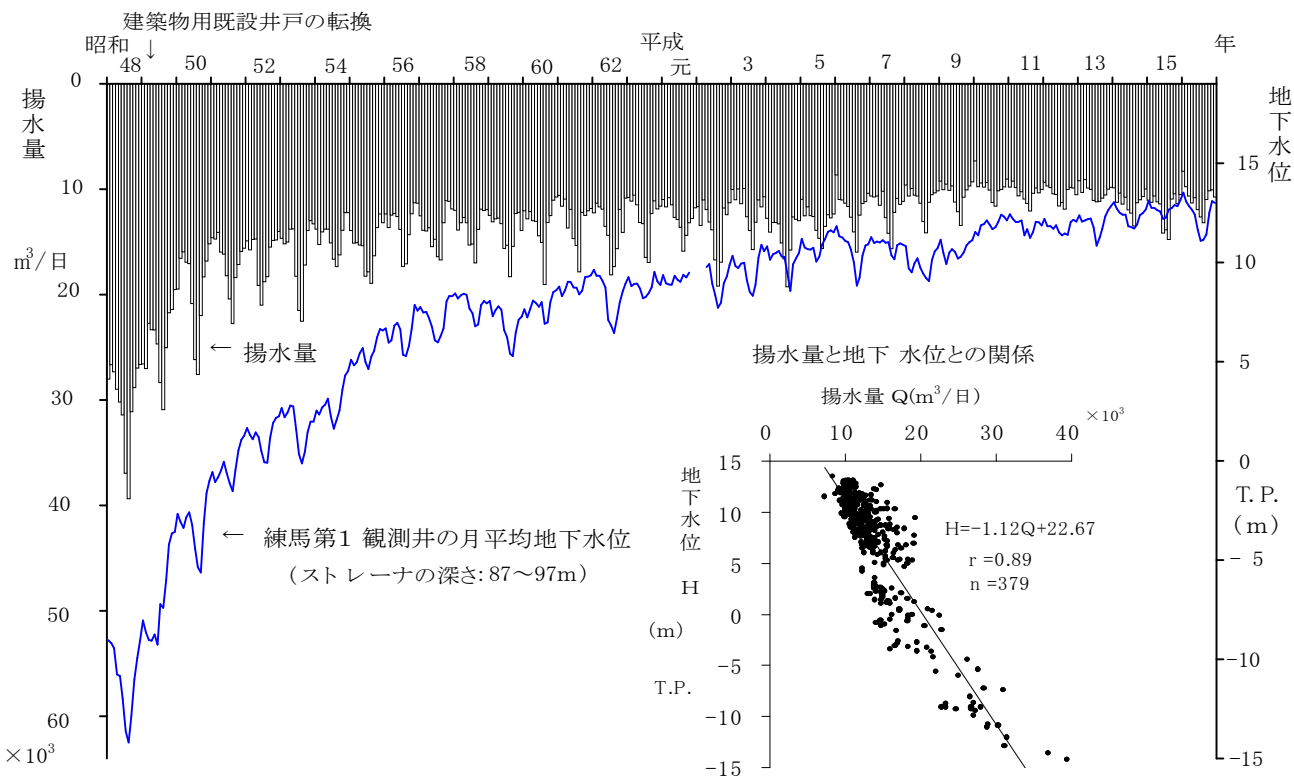
図-21 練馬区内の揚水量と地下水位の関係
