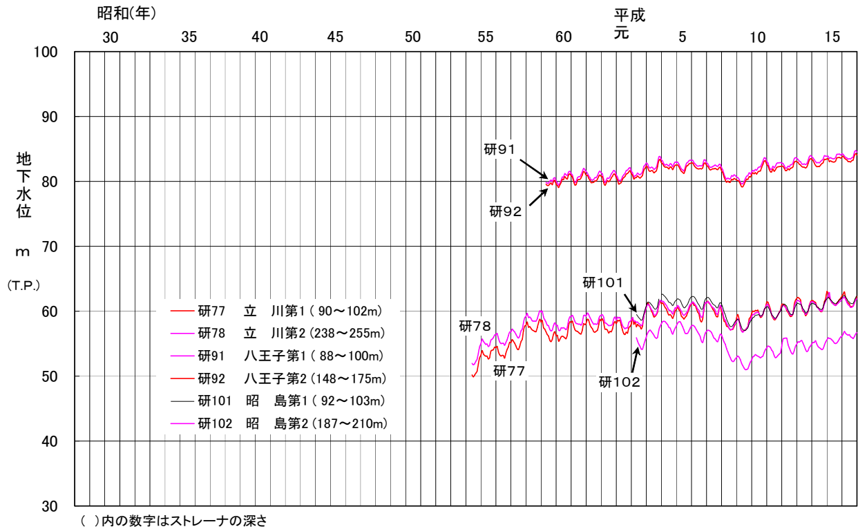
図-19 観測井の地下水水位変動図 (立川市、八王子市、昭島市)
