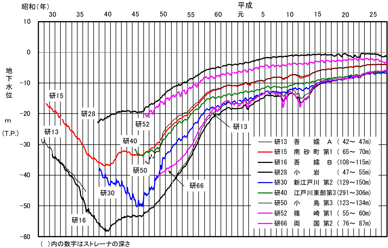
図-5 主な観測井の地下水水位変動図（江東区、墨田区、江戸川区）
