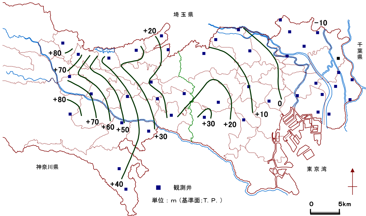
図-3 平成27年末の地下水位等高線図
