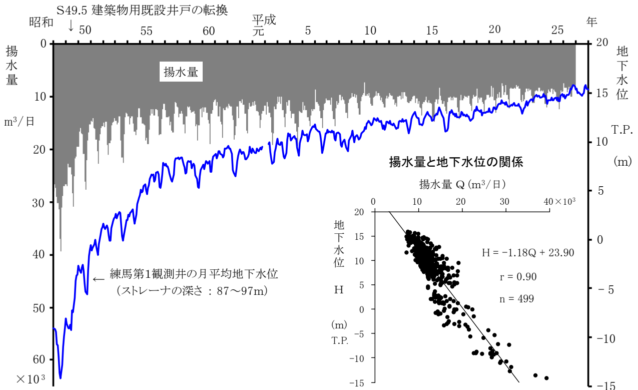
図-12 練馬区内の揚水量と地下水水位との関係
