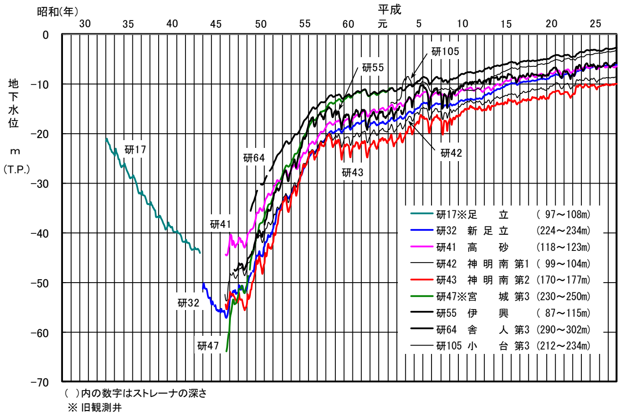
図-6 主な観測井の地下水水位変動図（足立区、葛飾区）
