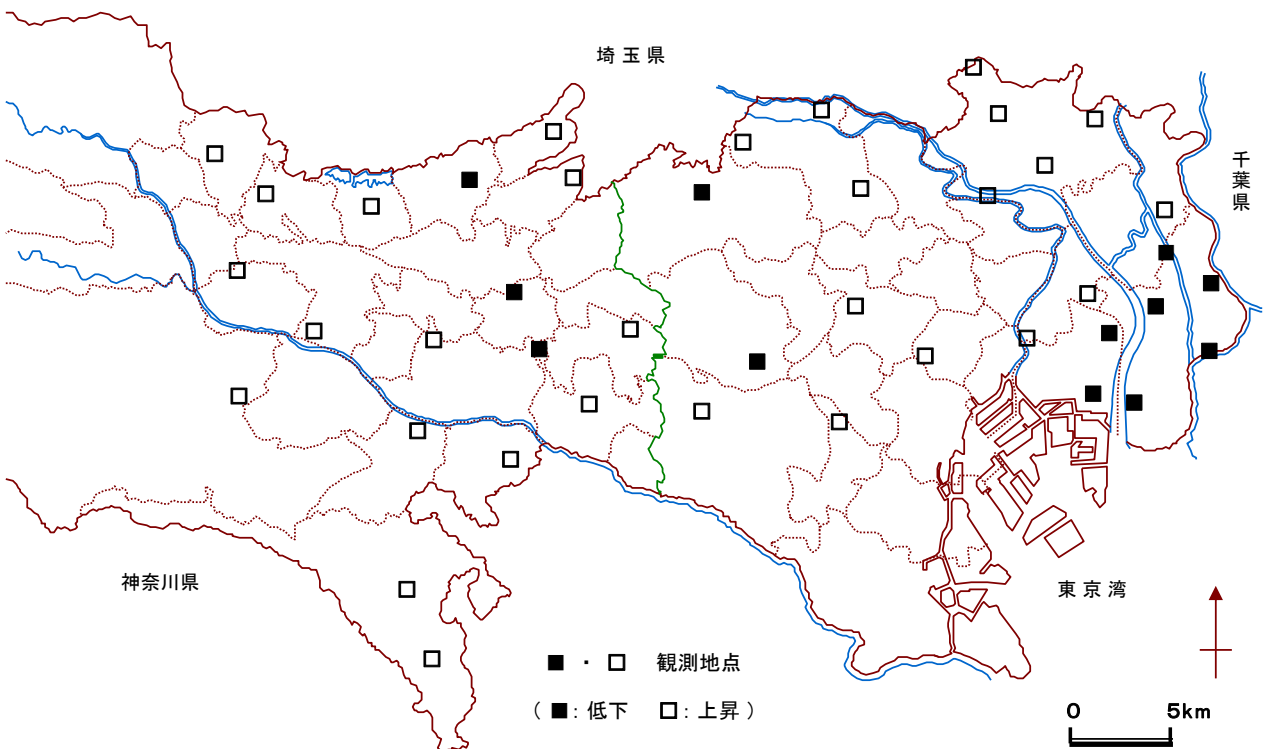
図-4 平成27年の地下水位変動状況図
