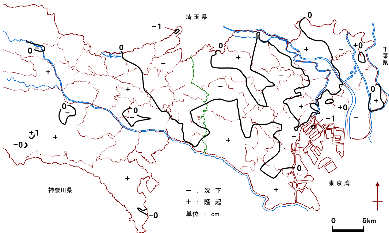
図-2 平成27年の地盤変動量図
