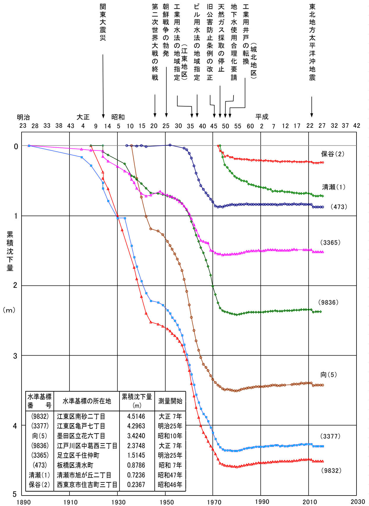
図-13 主要水準基標の累積沈下量図
