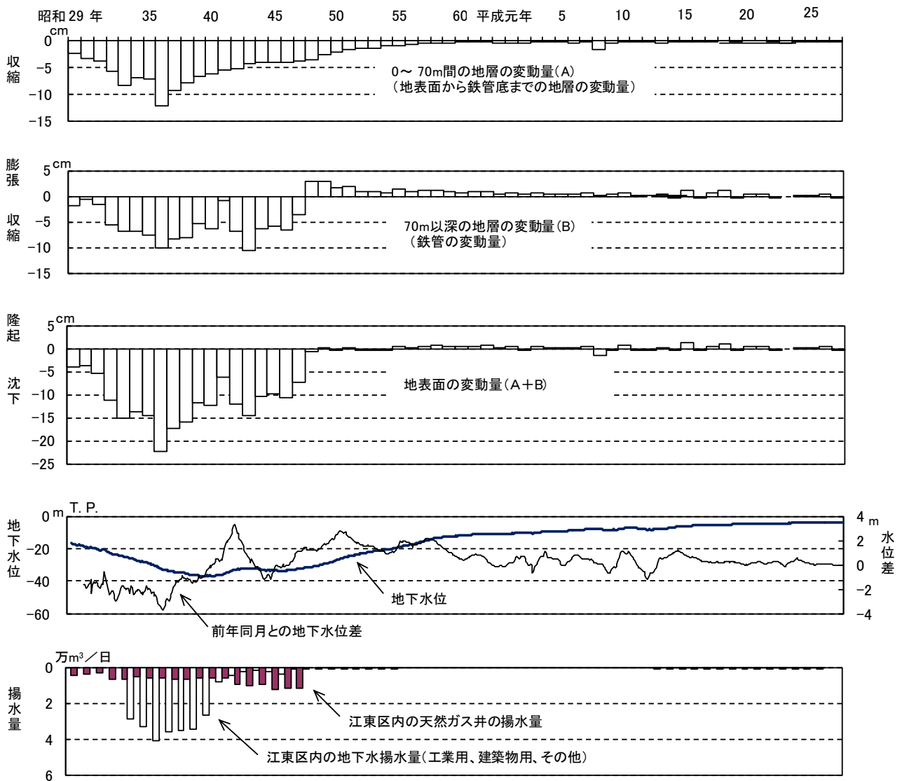
図-15 南砂町第1観測井(70m井)における地盤変動量と地下水位との関係
