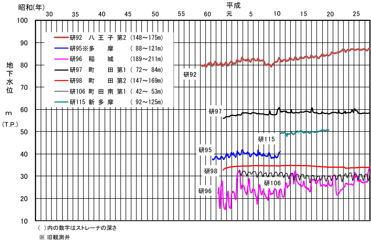
図-11 主な観測井の地下水水位変動図（八王子市、多摩市、稲城市、町田市）
