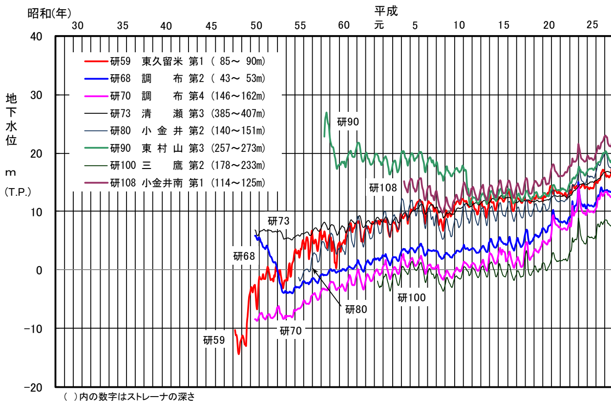
図-9 主な観測井の地下水位変動図（東久留米市、清瀬市、東村山市、小金井市、調布市、三鷹市）
