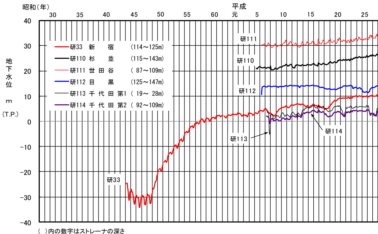
図-8 主な観測井の地下水位変動図（新宿区、杉並区、世田谷区、目黒区、千代田区）
