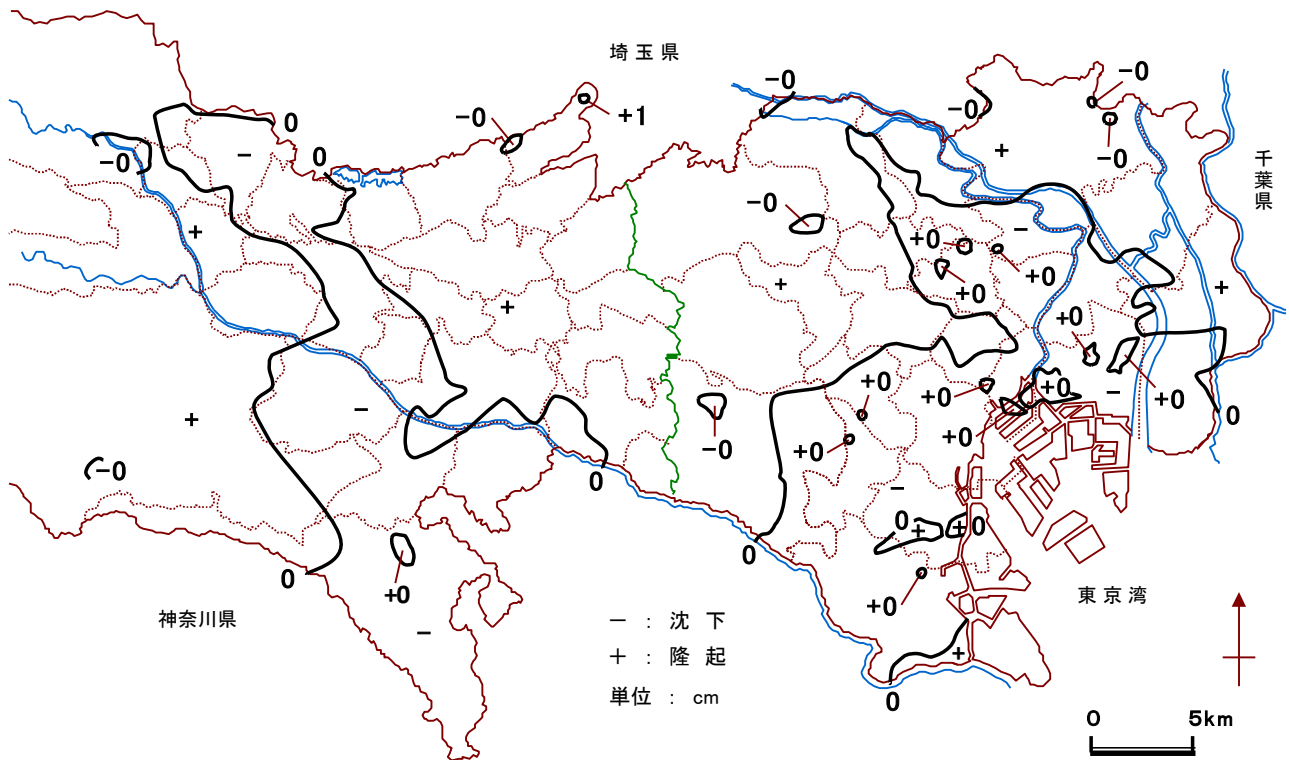
図-2 平成29年の地盤変動量図
