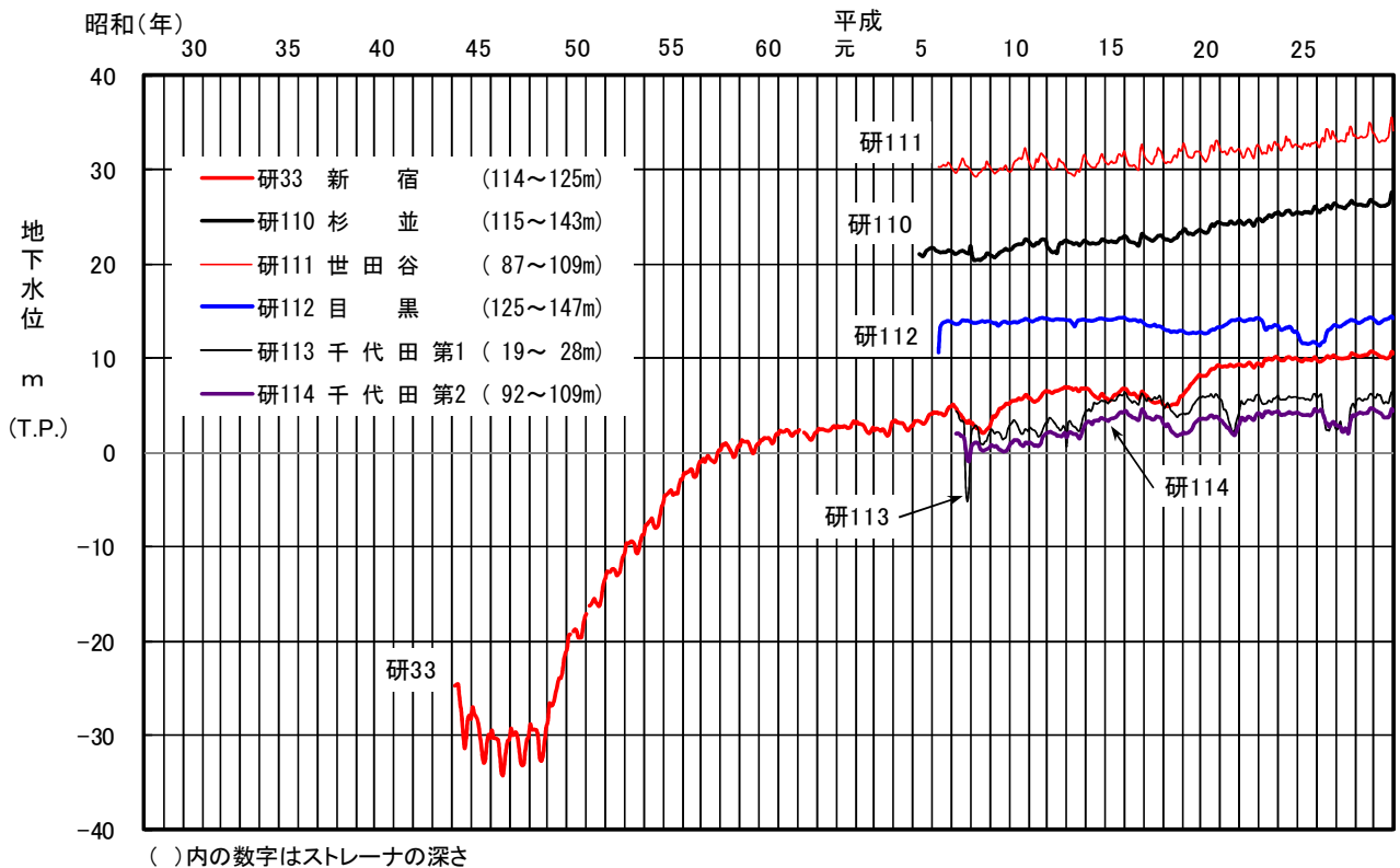
図-9 主な観測井の地下水位変動図 (新宿区、杉並区、世田谷区、目黒区、千代田区)
