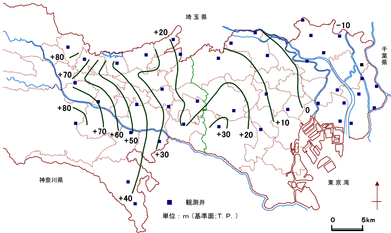
図-4 平成29年末の地下水位等高線図
