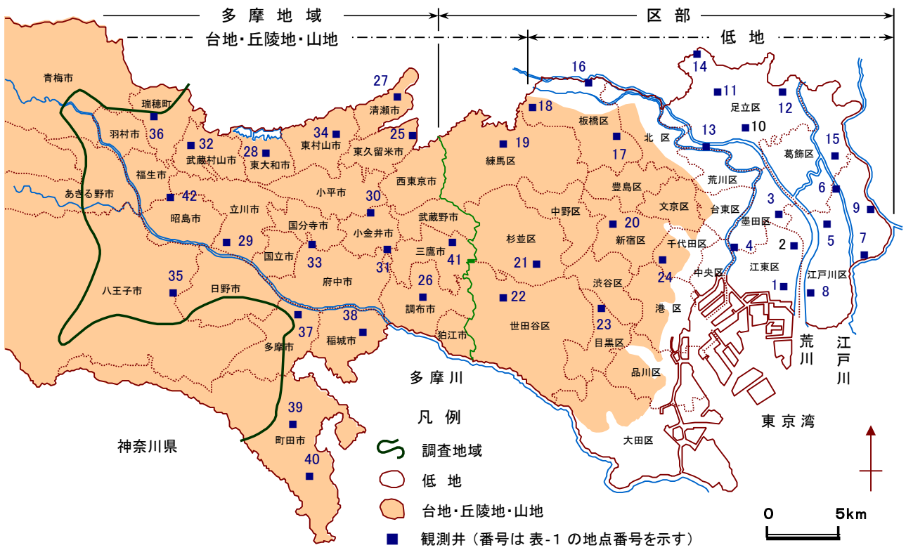
図-1 調査地域と観測井配置図
