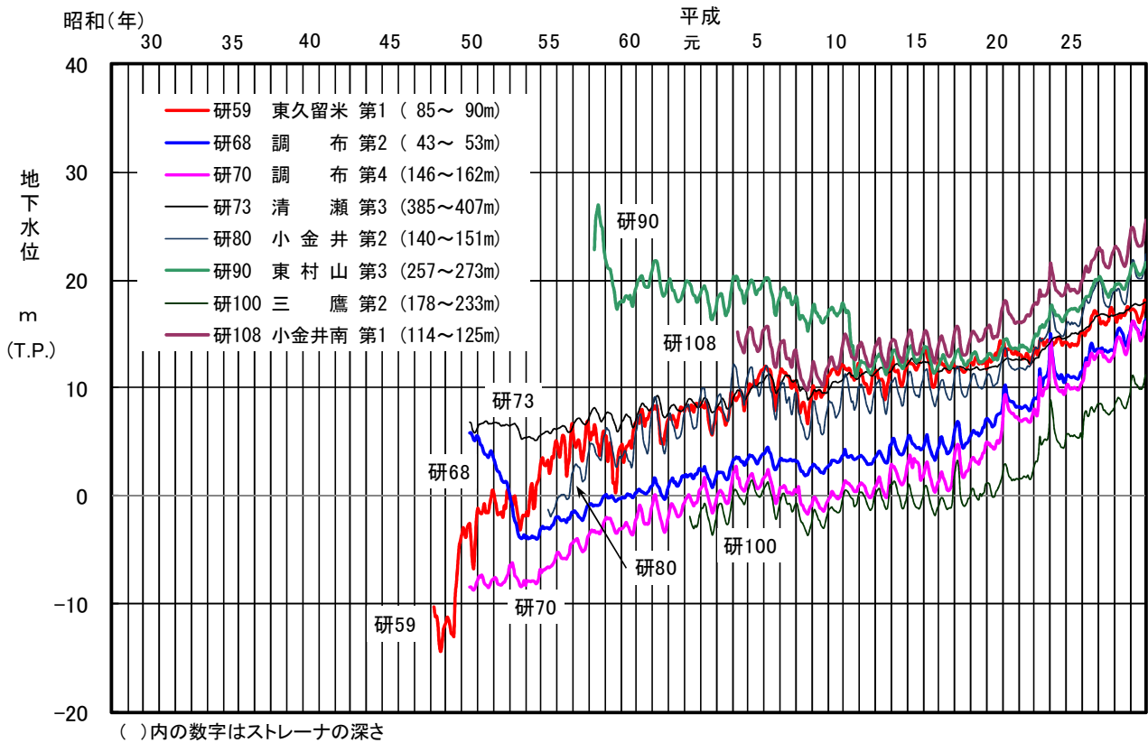
図-10 主な観測井の地下水位変動図（東久留米市、清瀬市、東村山市、小金井市、調布市、三鷹市）
