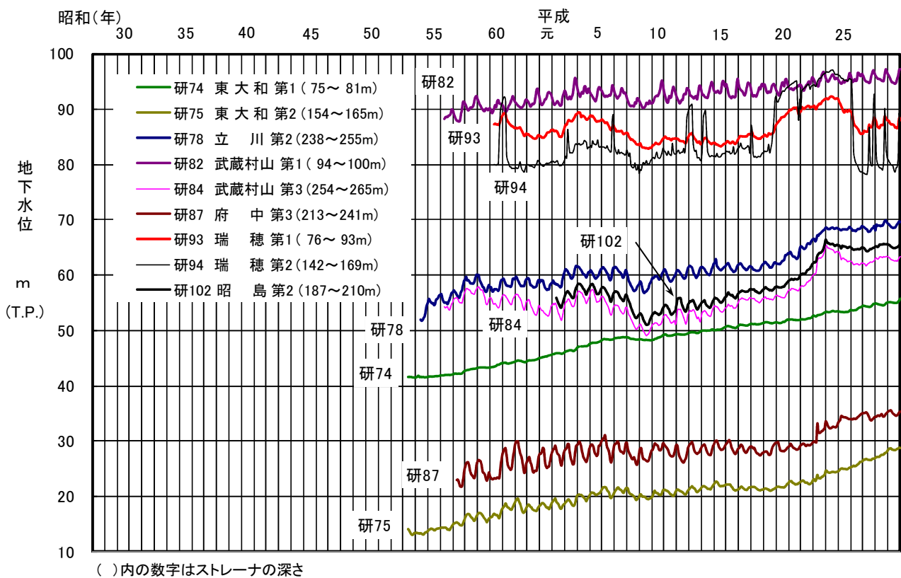
図-11 主な観測井の地下水位変動図（東大和市、武蔵村山市、瑞穂町、昭島市、立川市、府中市）
