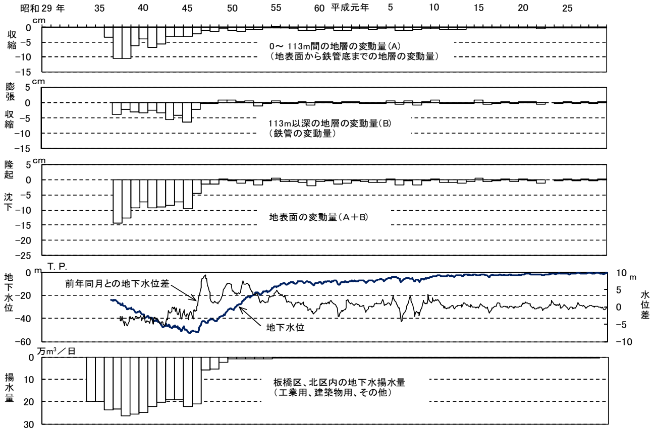
図-17 戸田橋第2観測井(113m井)における地盤変動量と地下水位との関係
