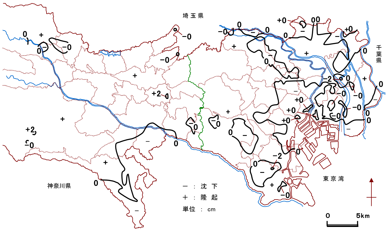
図-3 最近5年間の地盤変動量図（平成25年～平成29年）
