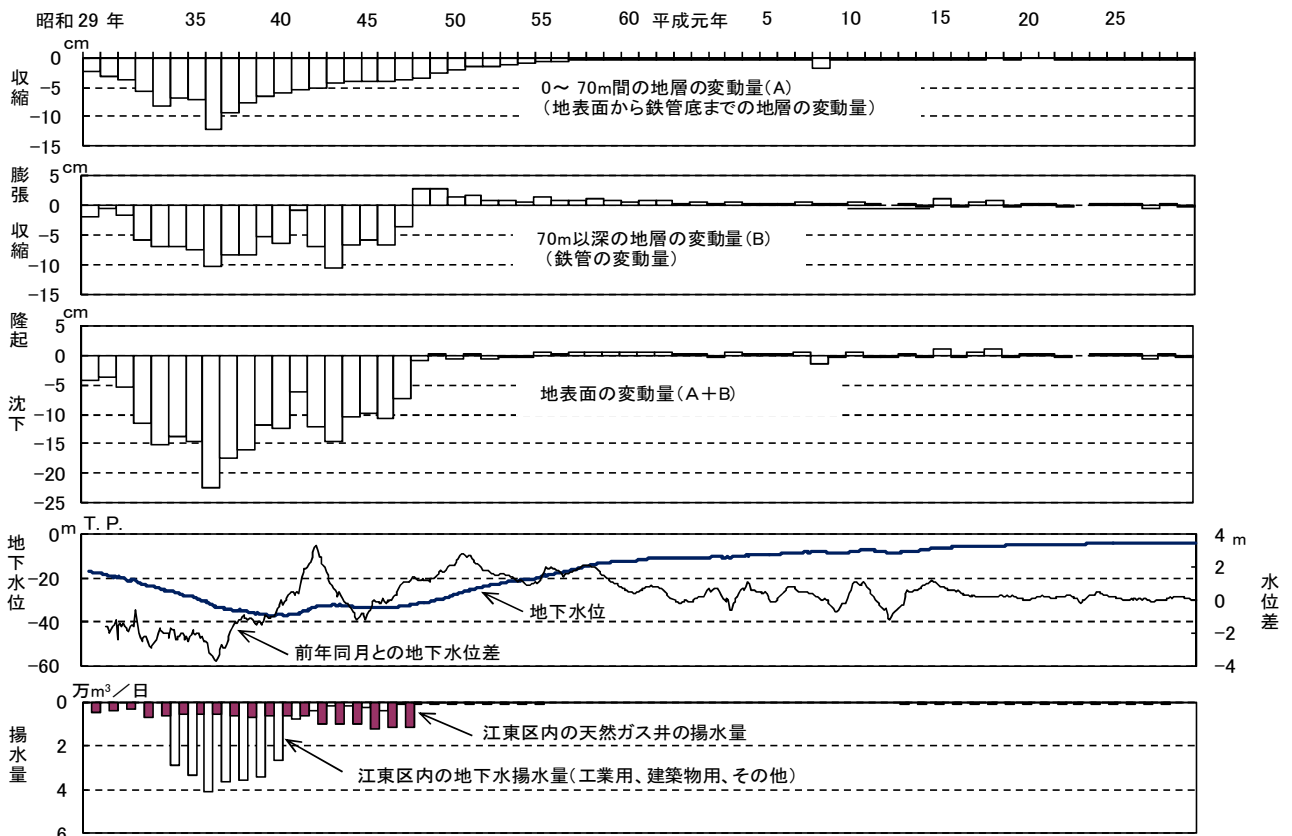
図-16 南砂町第1観測井(70m井)における地盤変動量と地下水位との関係
