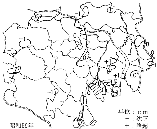
図-15 区部の地盤変動状況の変遷
