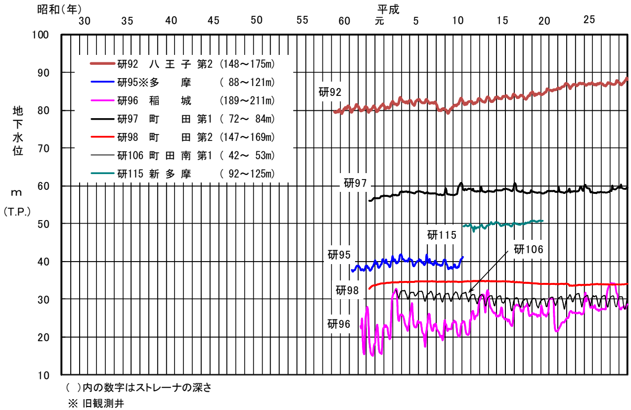
図-12 主な観測井の地下水位変動図（八王子市、多摩市、稲城市、町田市）
