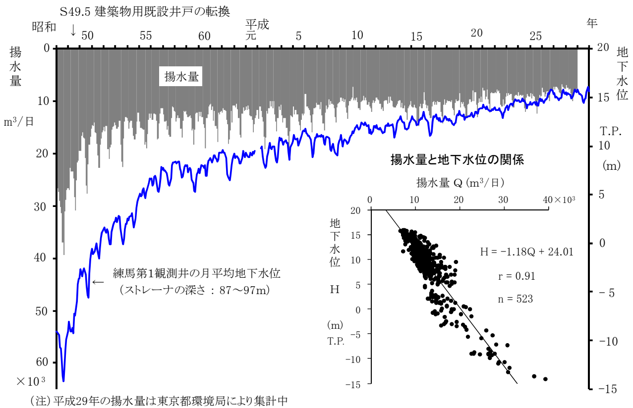
図-13 練馬区内の揚水量と地下水位との関係
