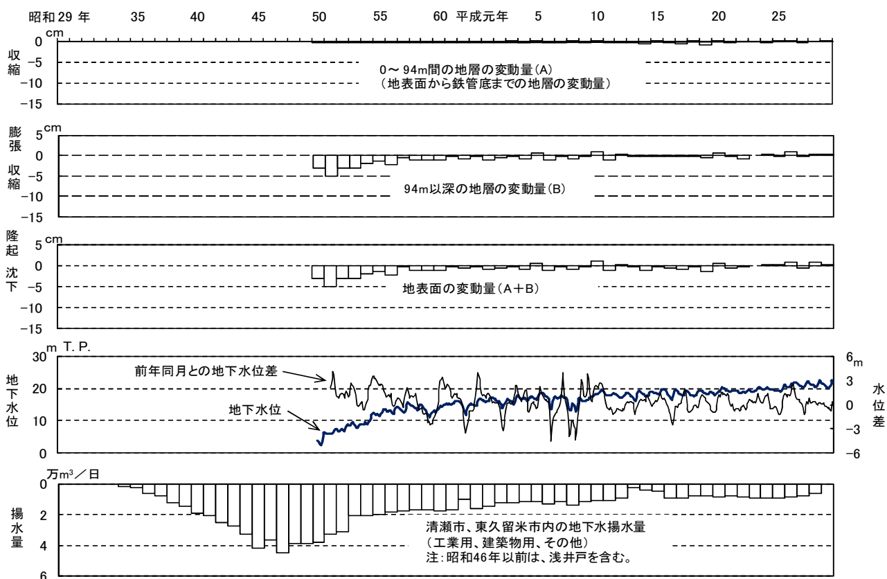
図-19 清瀬第1観測井(94m井)における地盤変動量と地下水位との関係
