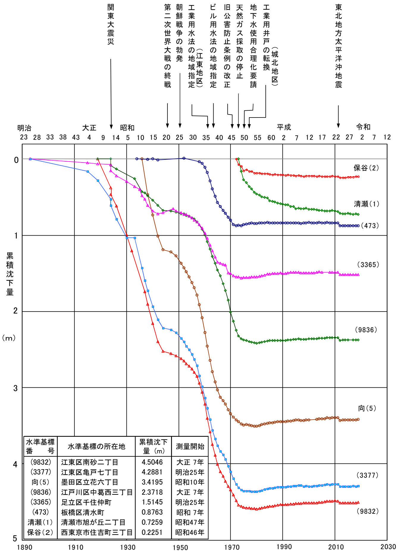
図-14 主要水準基標の累積沈下量図
