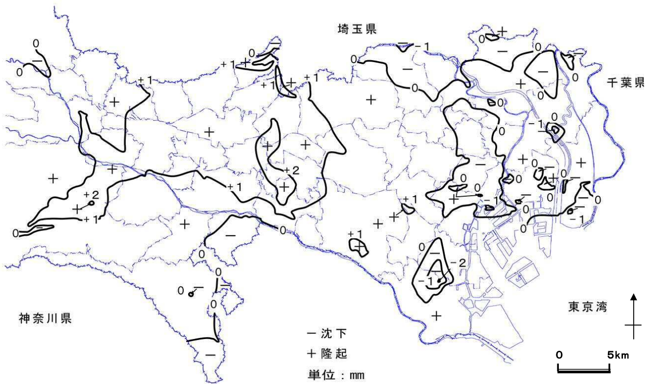
図-3 最近5年間の地盤変動量図（平成26年～平成30年）
