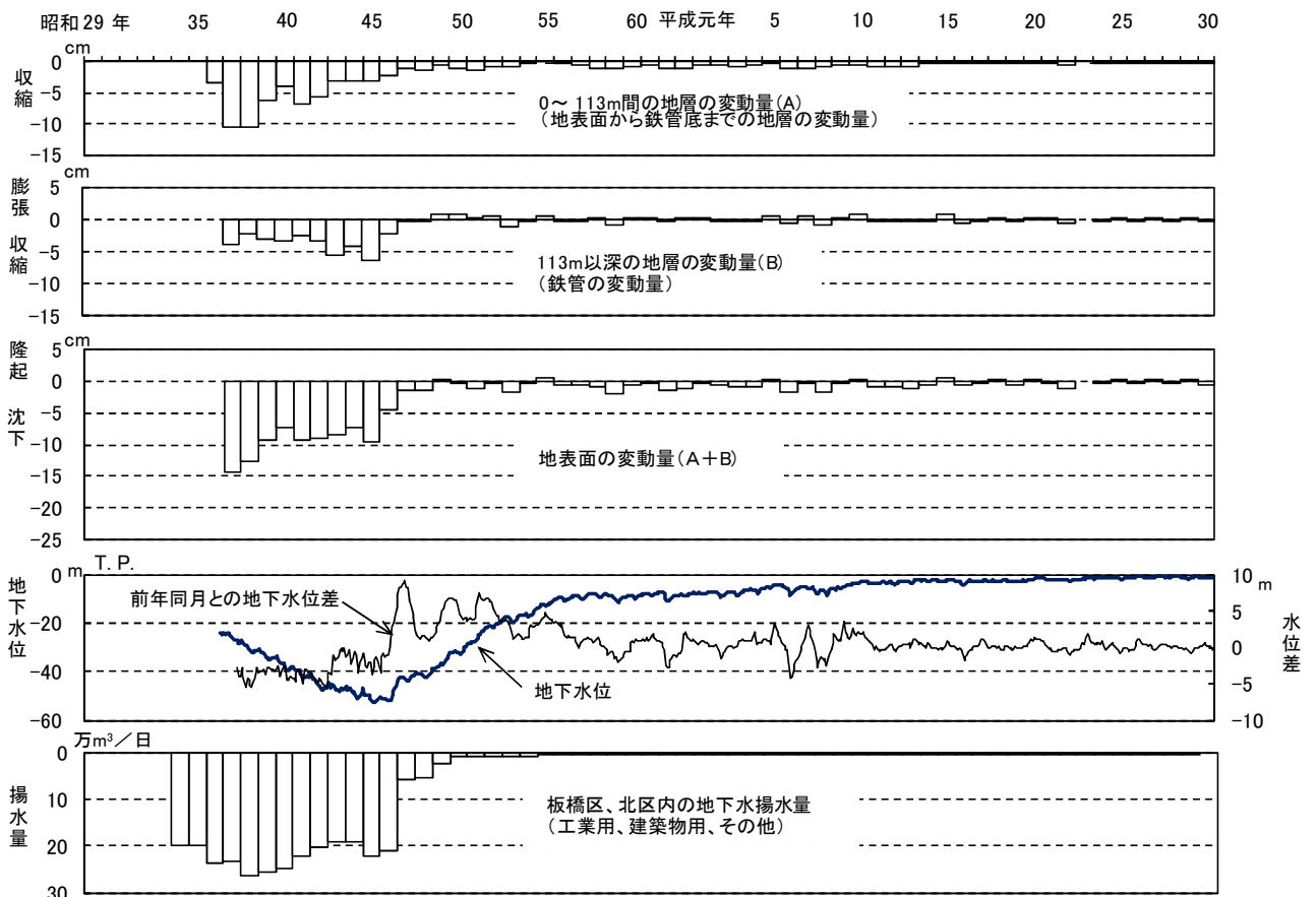
図-17 戸田橋第2観測井(113m井)における地盤変動量と地下水水位との関係
