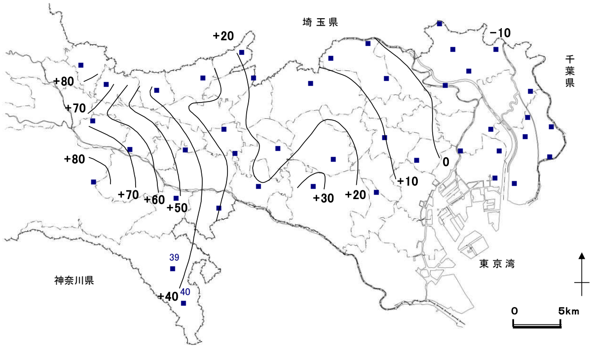
図-4 平成30年末の地下水位等高線図
