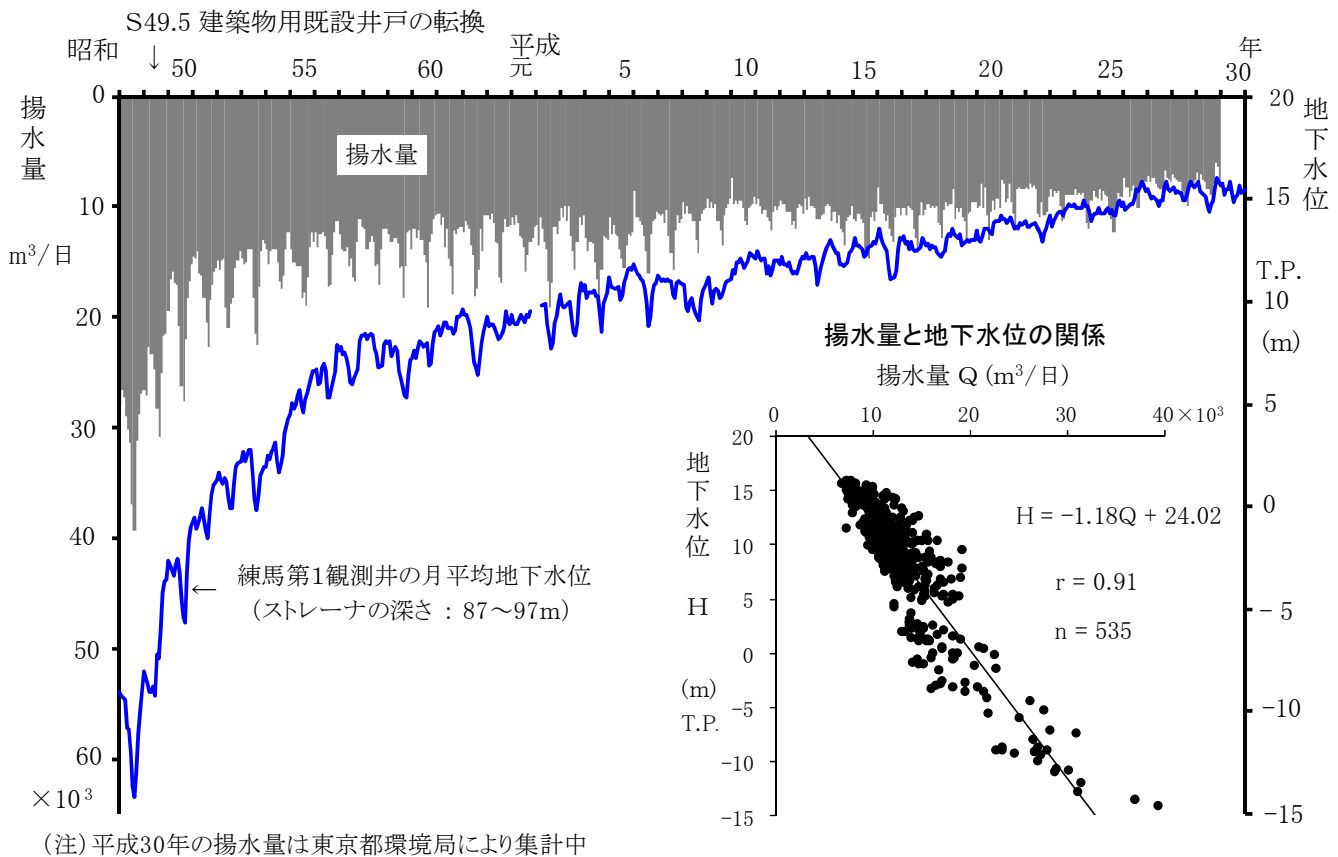
図-13 練馬区内の揚水量と地下水水位との関係
