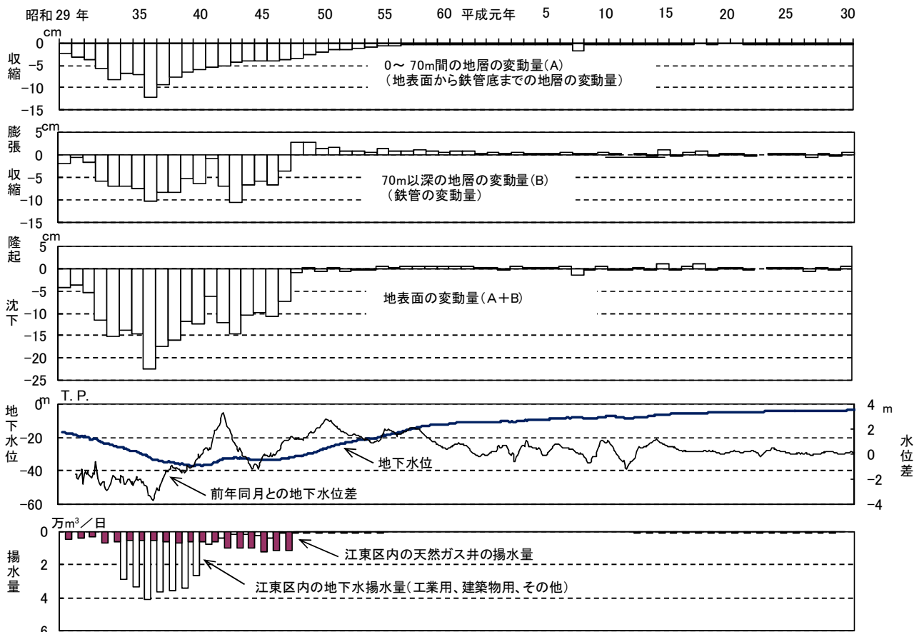
図-16 南砂町第1観測井(70m井)における地盤変動量と地下水水位との関係
