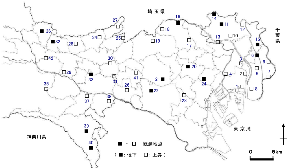
図-5 平成30年の地下水位変動状況図 (番号は表-1の地点番号を示す)
