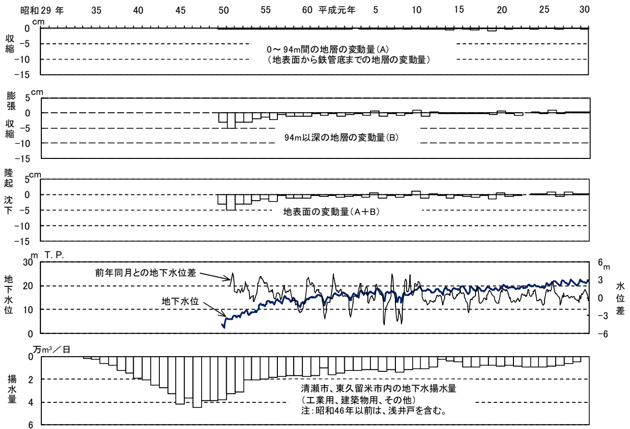
図-19 清瀬第1観測井(94m井)における地盤変動量と地下水水位との関係
